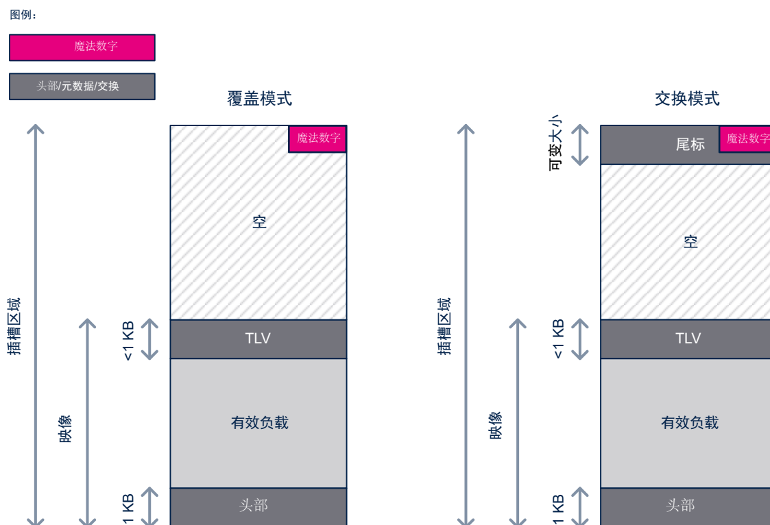
图 17. 固件映像和插槽区域
