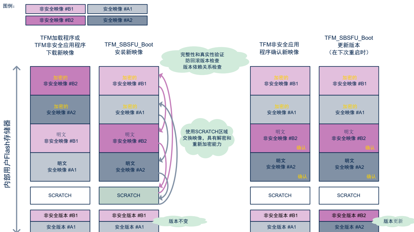
图 15. 交换模式的新固件下载和安装流程（有映像确认）
