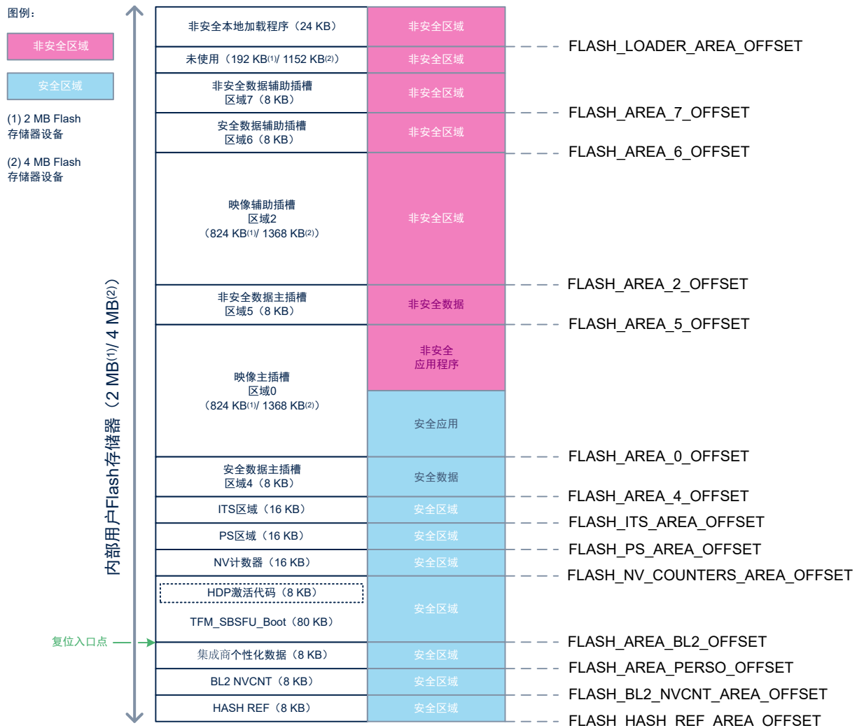
图 9. STM32U5 TFM Flash 存储器布局（一个映像）
