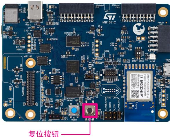
图 50. 复位按钮 B-U585I-IOT02A
