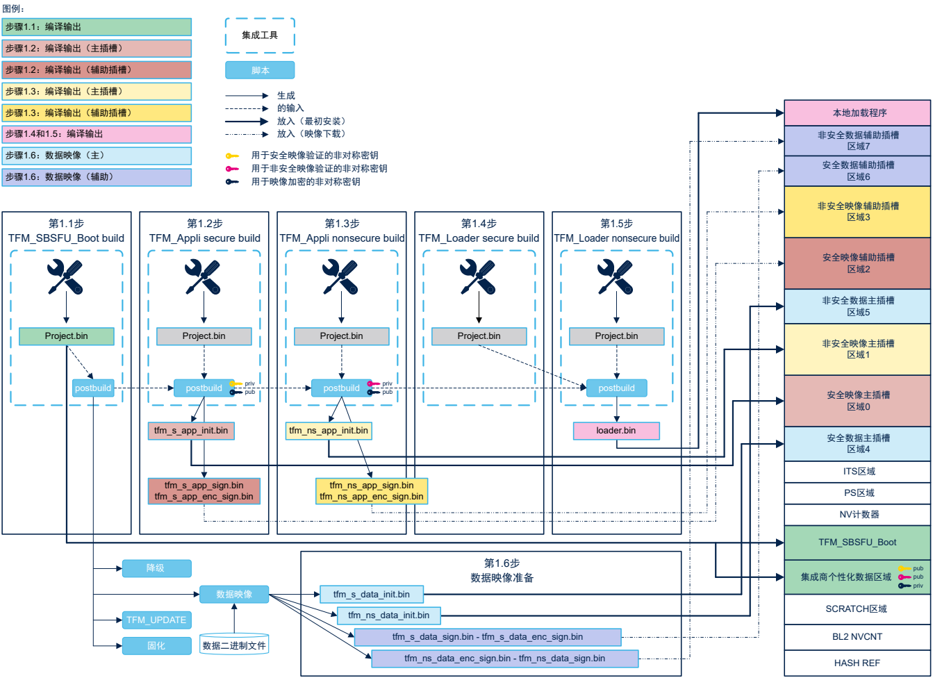
图 25. 编译过程概述
