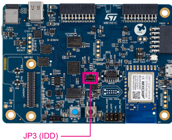
图 52. B-U585I-IOT02A 板上要移除的跳线
