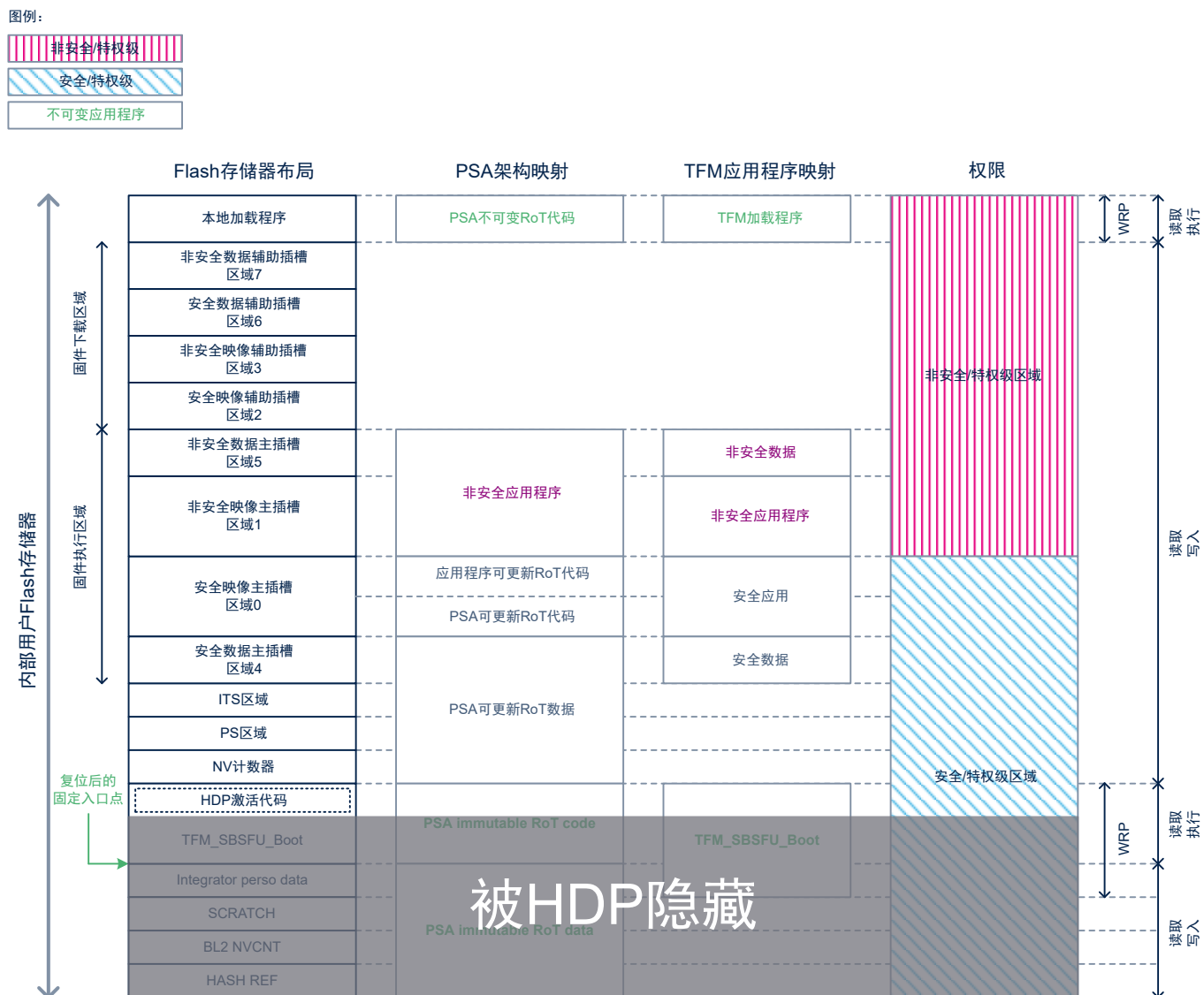
图 76. Flash 离开 TFM_SBSFU_Boot 应用程序前往非安全本地加载程序时的保护措施总览
