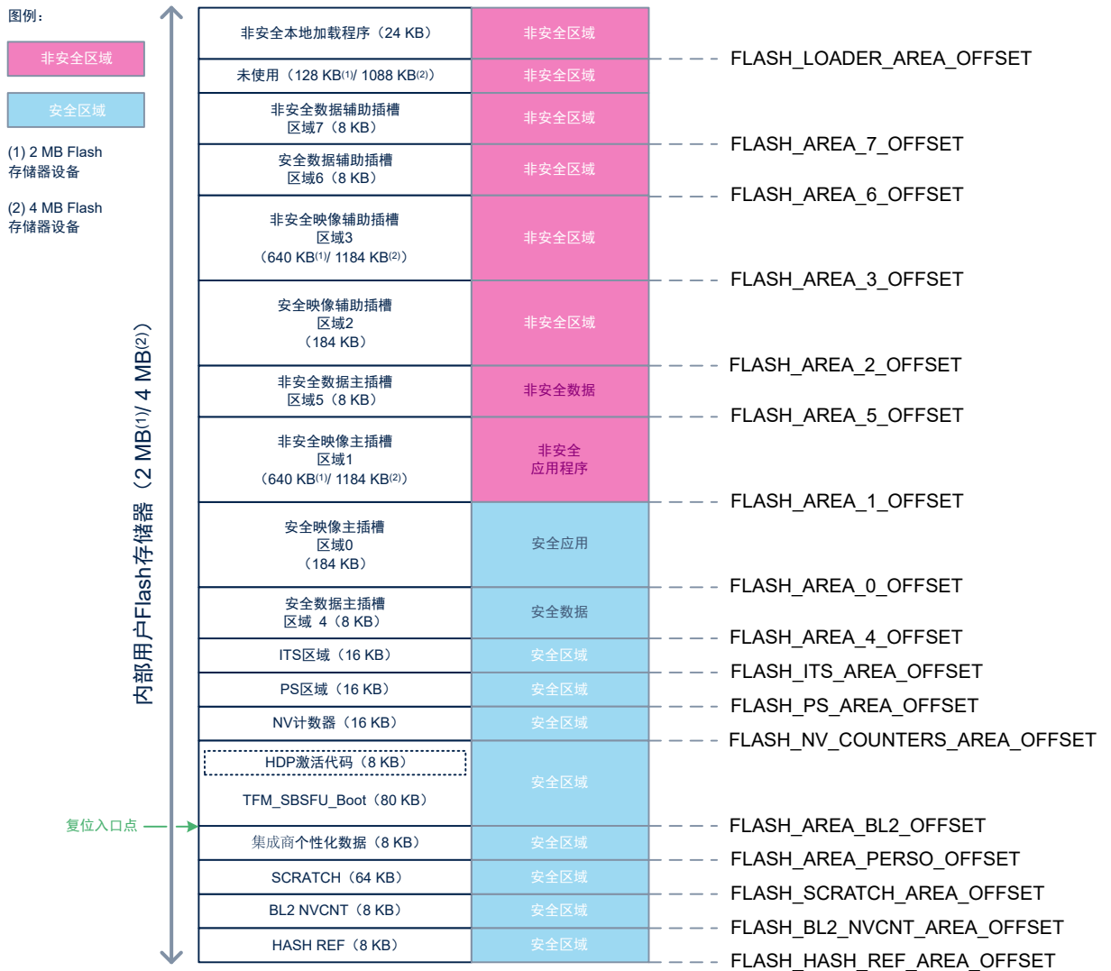
图 10. STM32U5 TFM Flash 存储器布局（交换模式）
