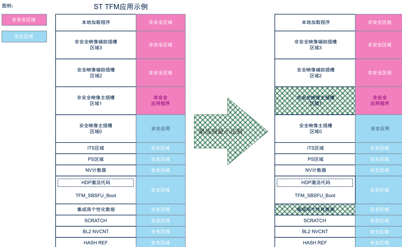
图 71. 集成商最小定制要求
