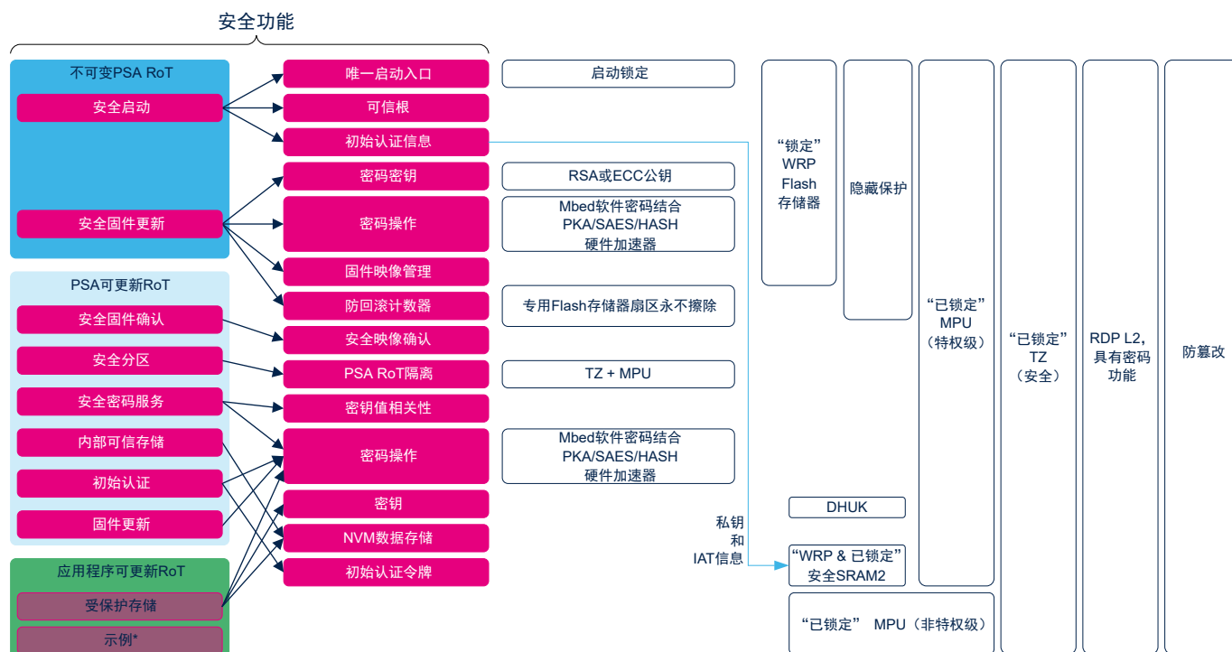
图 4. 使用 STM32U5 安全外设的 TFM 应用程序
