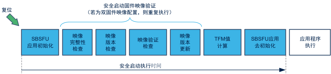
图 79. 安全启动执行时间
