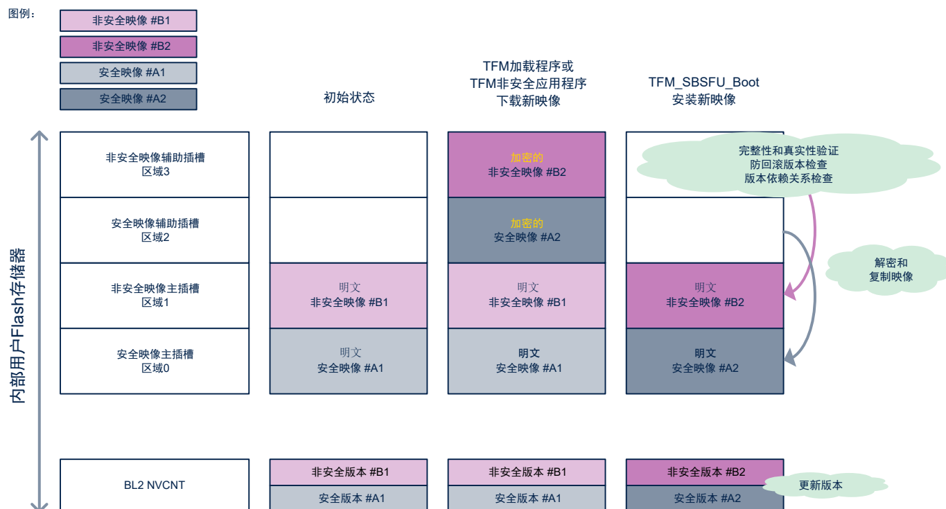
图 11. 双固件映像配置以及主和辅助插槽配置下覆盖模式的新固件下载和安装流程
