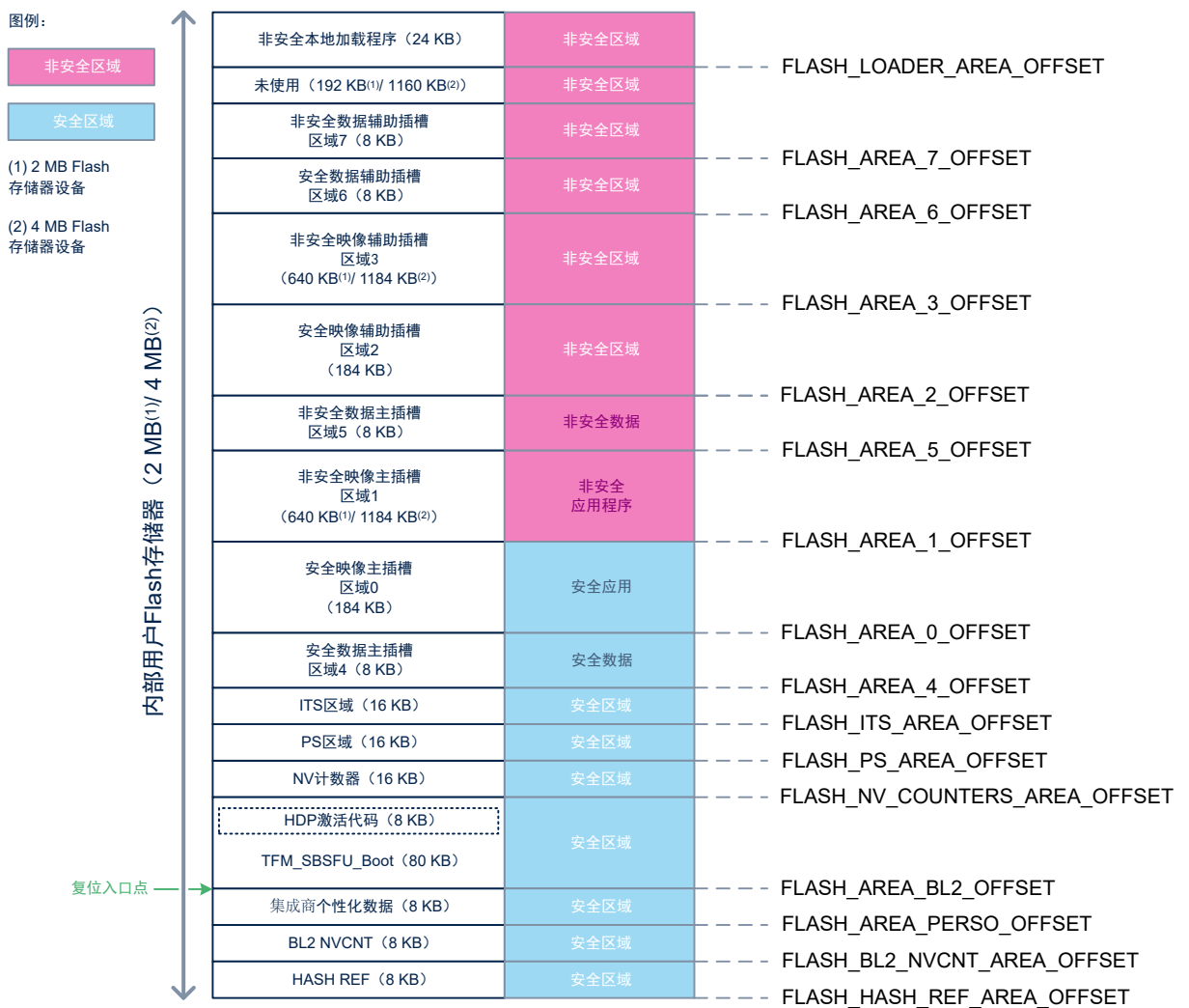
图 7. STM32U5 TFM Flash 存储器布局（默认配置）
