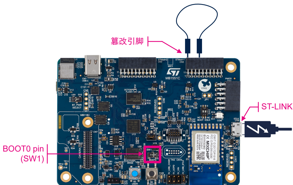
图 23. B-U585I-IOT02A 开发板设置
