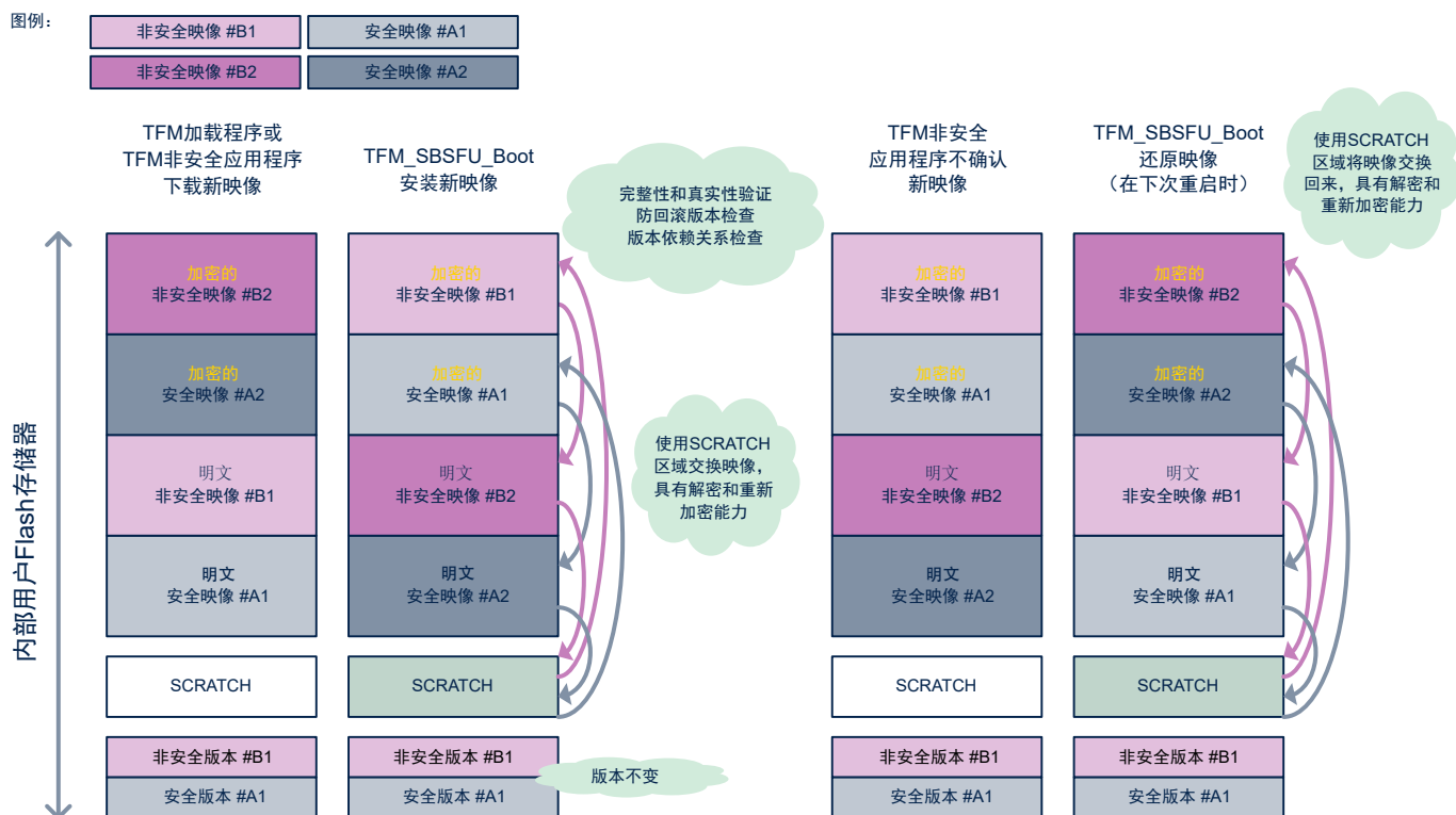
图 16. 交换模式的新固件下载和安装流程（无映像确认）
