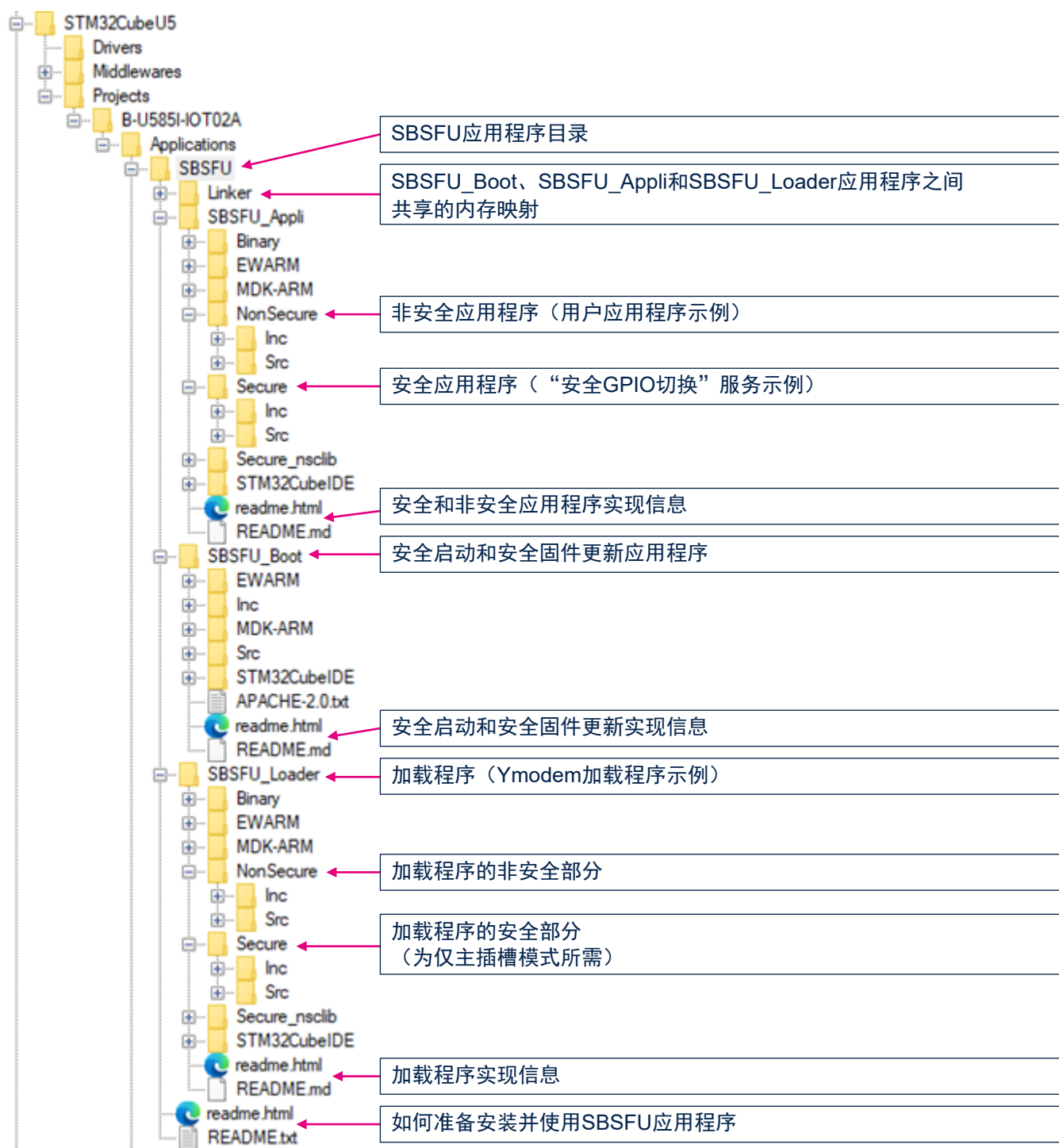
图 21. 项目文件夹结构 (2/3)
