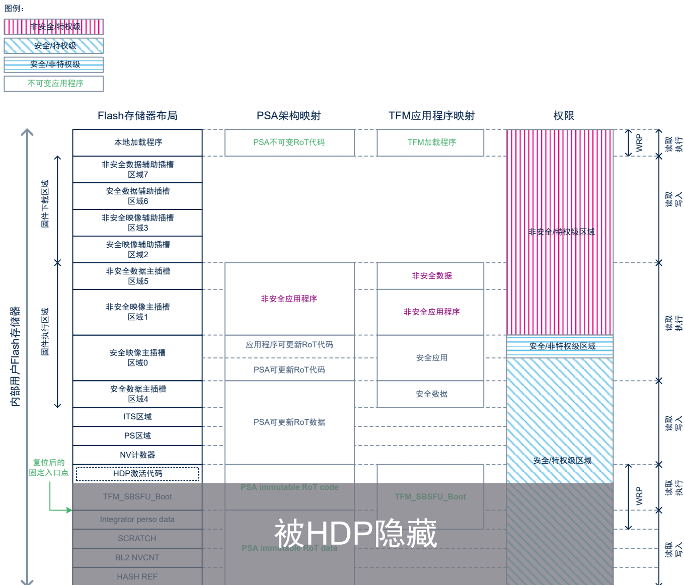
图 75. Flash 应用程序执行期间的 Flash 存储器保护措施总览
