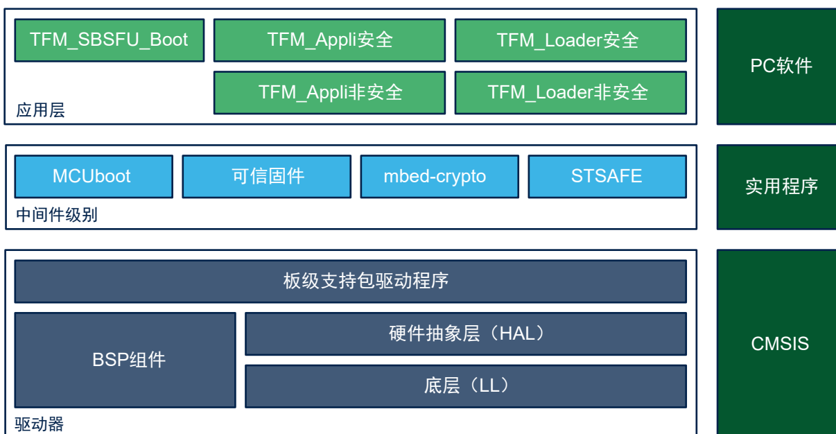
图 6. TFM 应用程序架构
