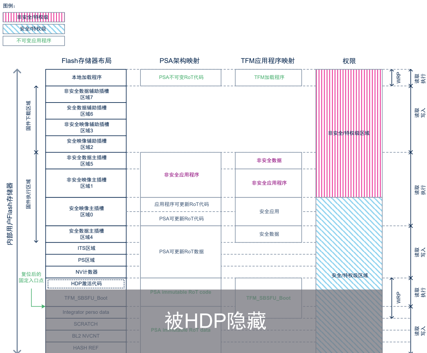
图 74. Flash 离开 TFM_SBSFU_Boot 应用程序前往 TFM 应用程序时的保护措施总览
