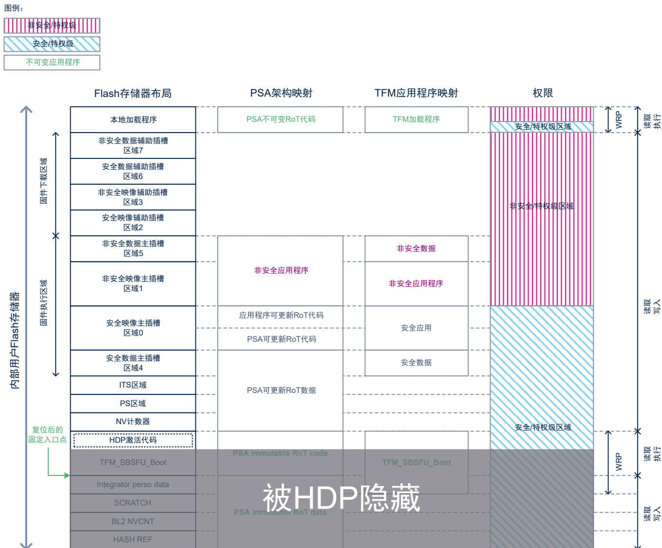
图 77. Flash 离开 TFM_SBSFU_Boot 应用程序前往安全和非安全本地加载程序时的保护措施总览
