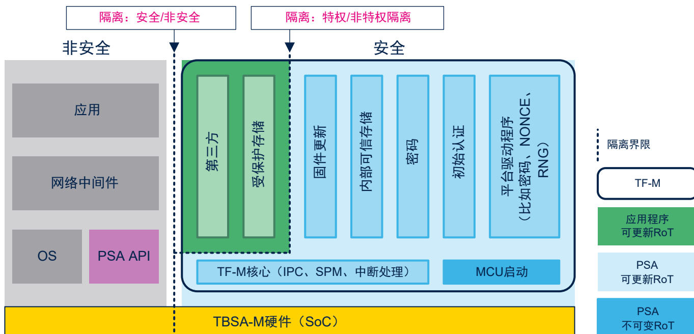
图 1. TF-M 概述
