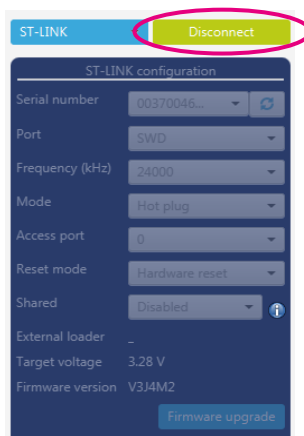
图 36. STM32CubeProgrammer 断开
