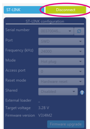
图 47. STM32CubeProgrammer 断开
