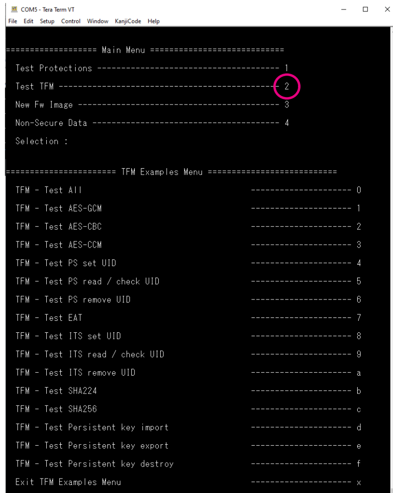
图 58. TFM 测试菜单
