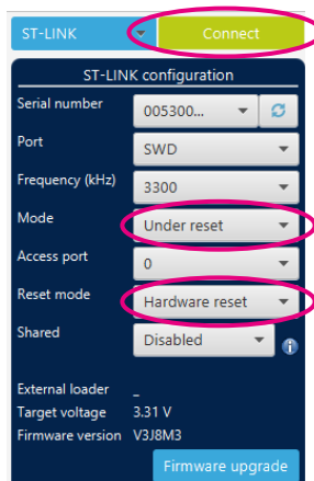
图 37. STM32CubeProgrammer 连接菜单
