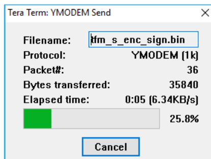
图 62. 正在进行固件映像传输
