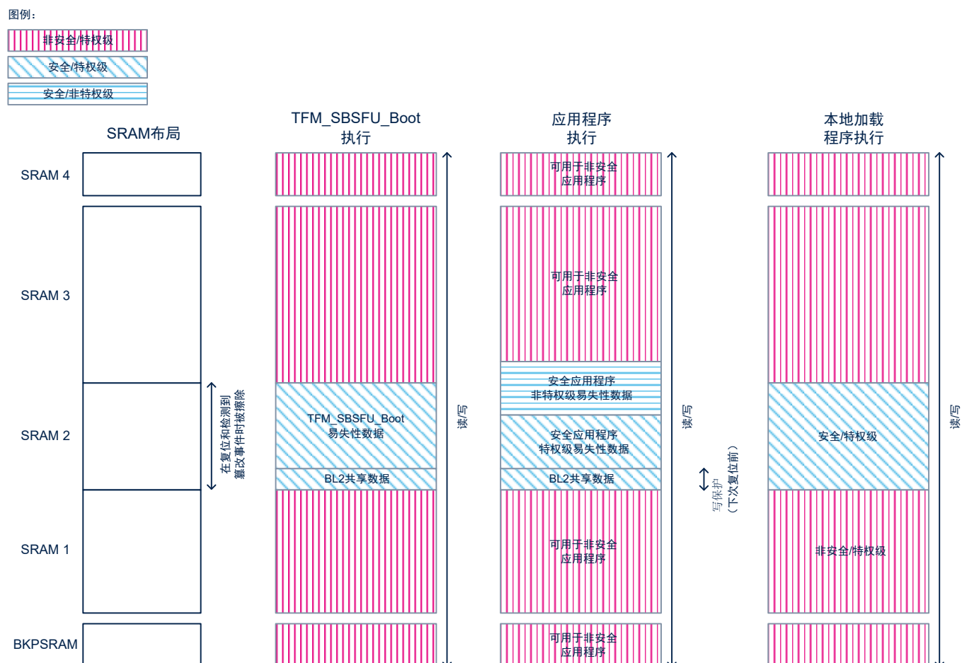
图 78. SRAM 保护功能概述
