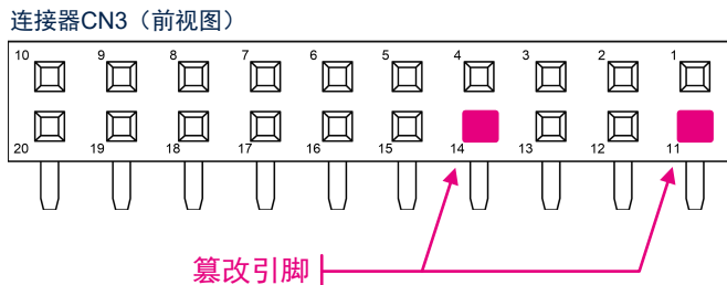
图 24. B-U585I-IOT02A 板设置（细部图）
