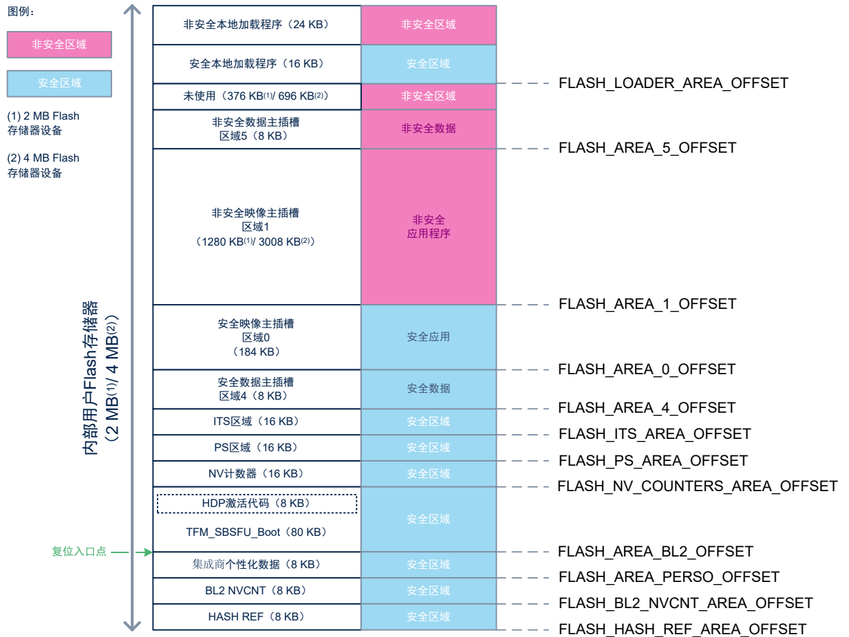
图 8. STM32U5 TFM Flash 存储器布局（仅主插槽）
