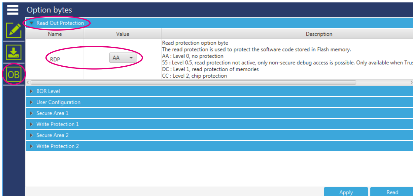
图 27. STM32CubeProgrammer 选项字节界面（读出保护）
