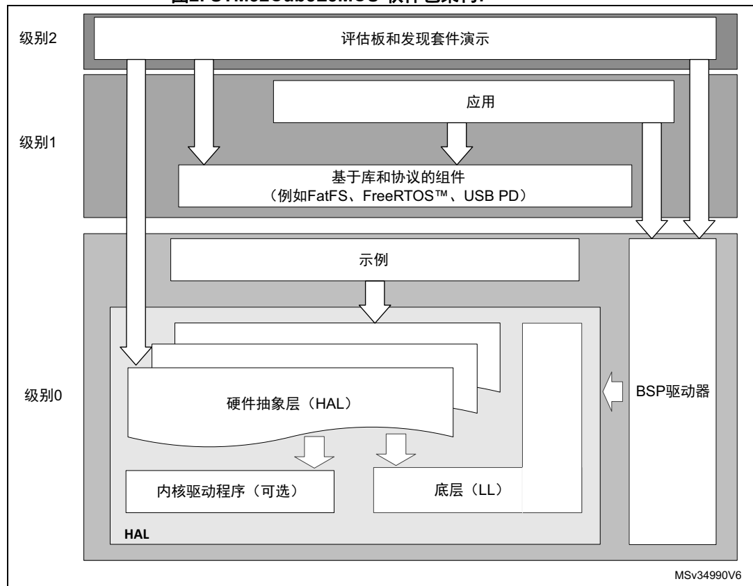
图2. STM32CubeL5 MCU 软件包架构7
