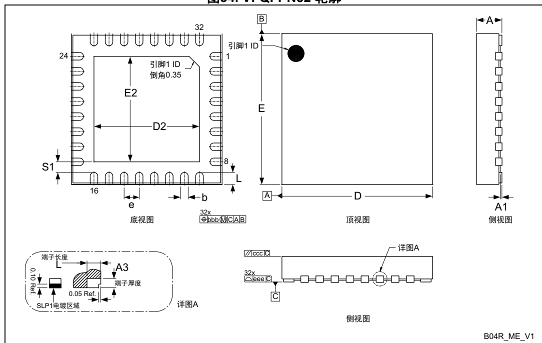
图34. VFQFPN32 轮廓
