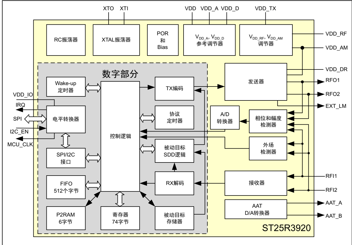
图3. ST25R3920框图
