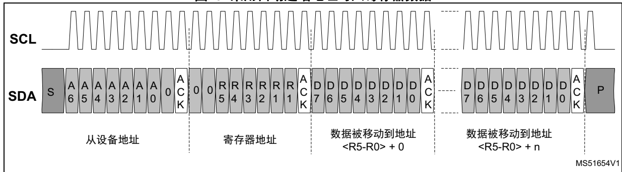
图19. 采用自动递增地址写入寄存器数据
