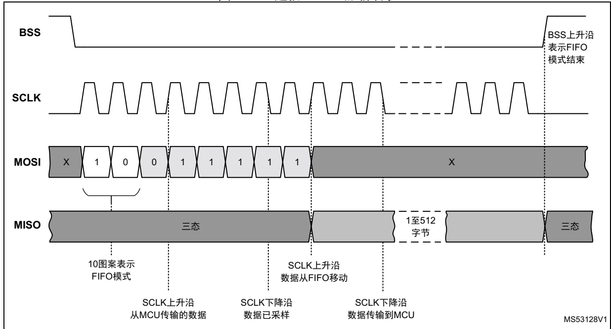
图15. SPI通信：FIFO加载读取
