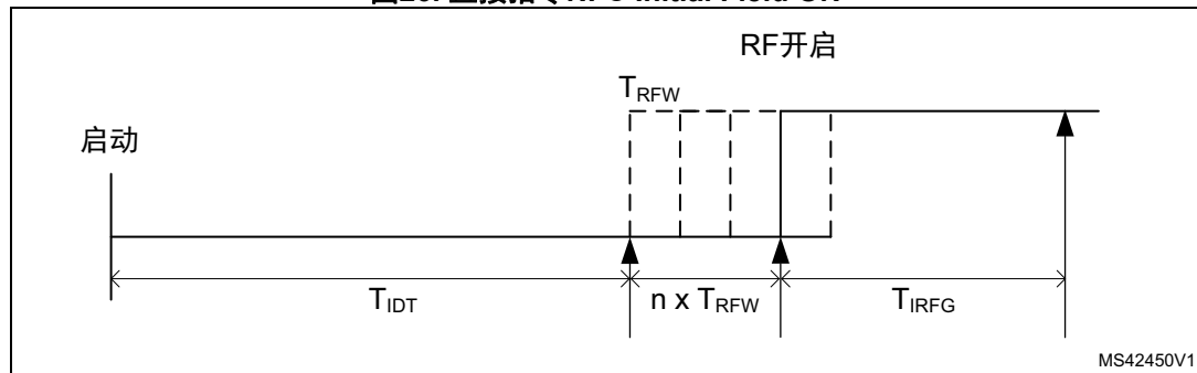
图26. 直接指令NFC Initial Field ON
