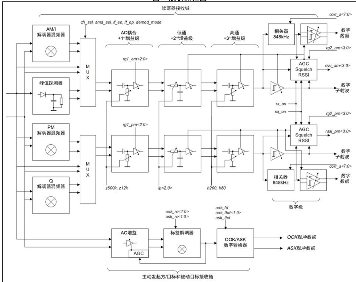
图5. 接收器框图
