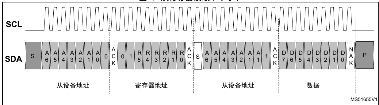
图20. 从寄存器读取单个字节
