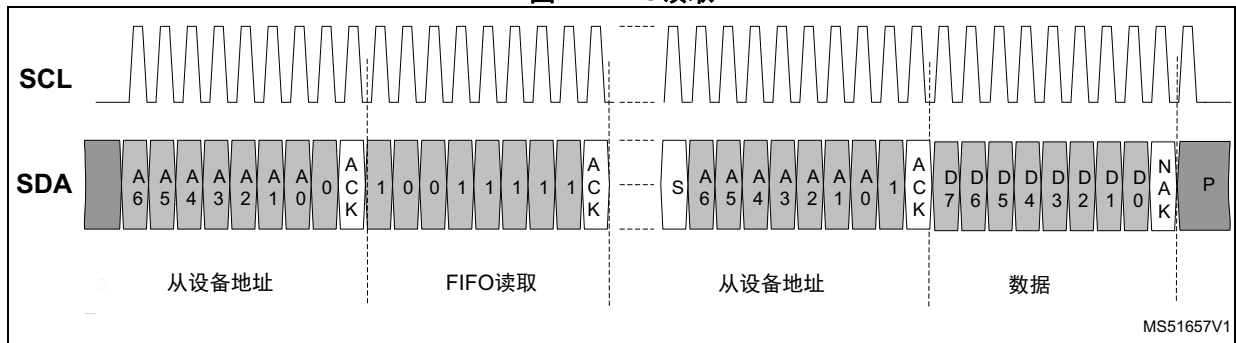
图22. FIFO读取
