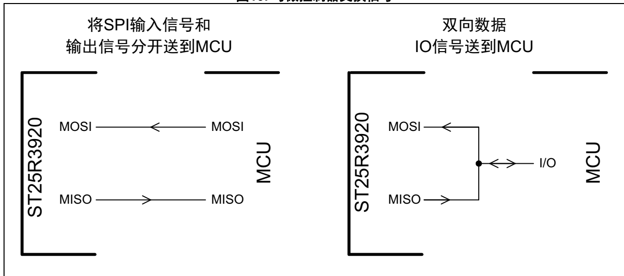
图10. 与微控制器交换信号
