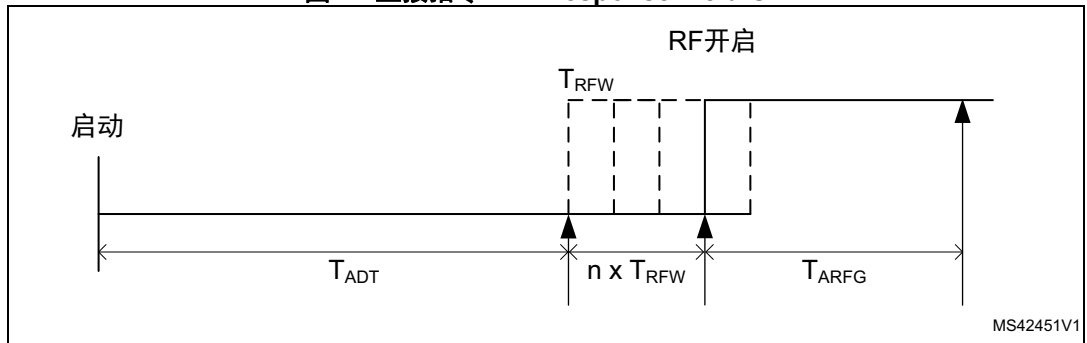
图27. 直接指令NFC Response Field ON
