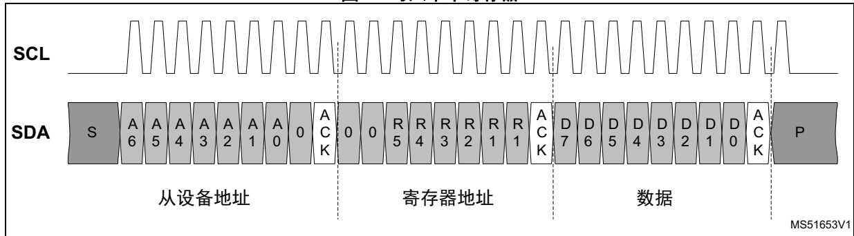
图18. 写入单个寄存器
