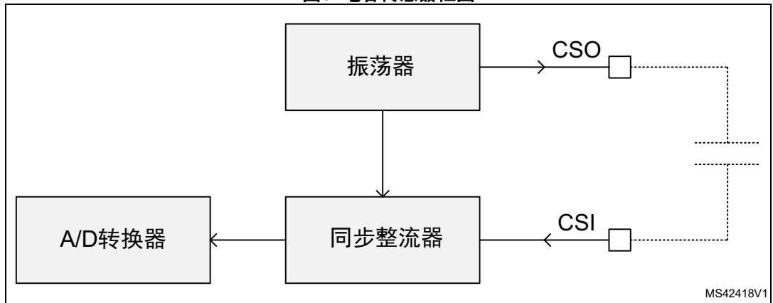
图6. 电容传感器框图
