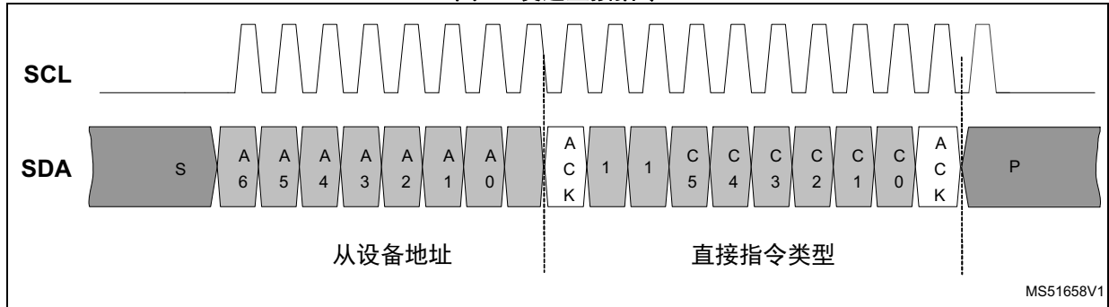
图23. 发送直接指令
