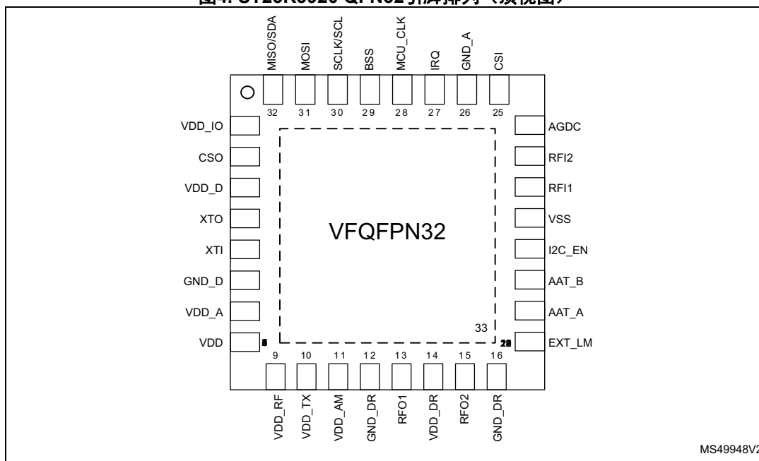
图4. ST25R3920 QFN32引脚排列（顶视图）
