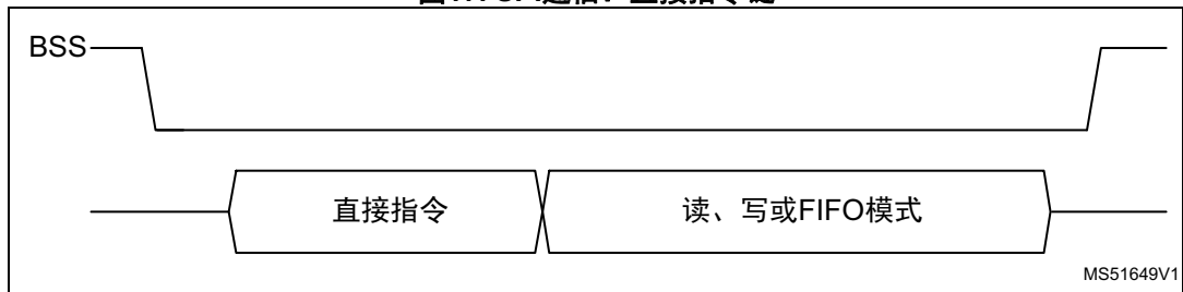
图17. SPI通信：直接指令链
