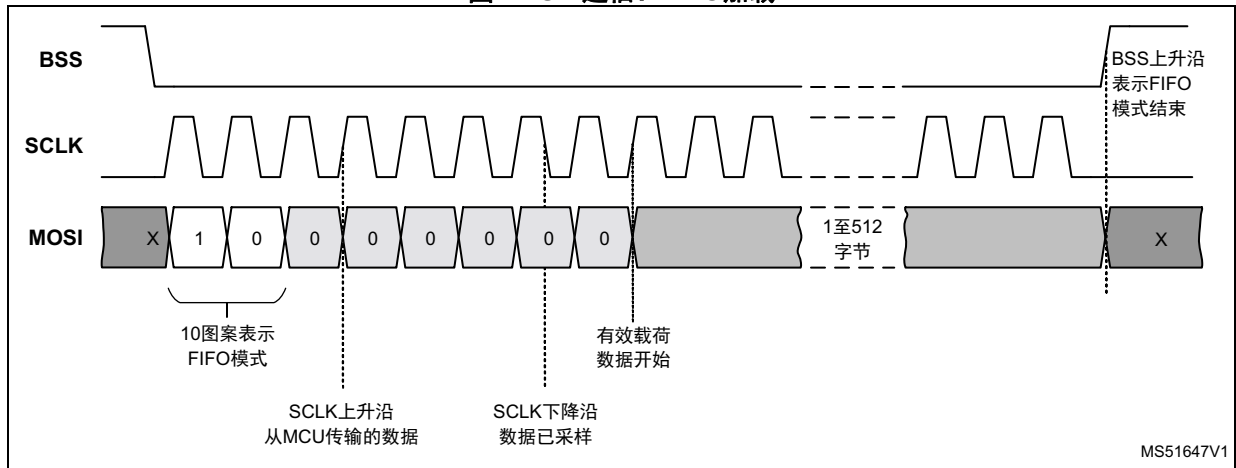
图14. SPI通信：FIFO加载
