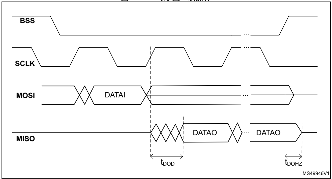
图29. SPI时序图 - 读操作
