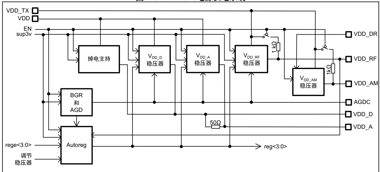
图9. ST25R3920电源供电系统
