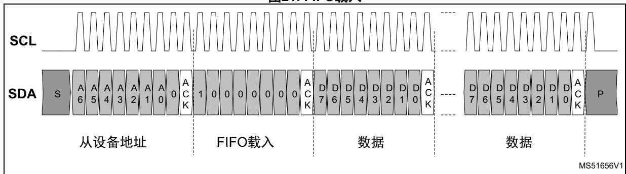
图21. FIFO载入
