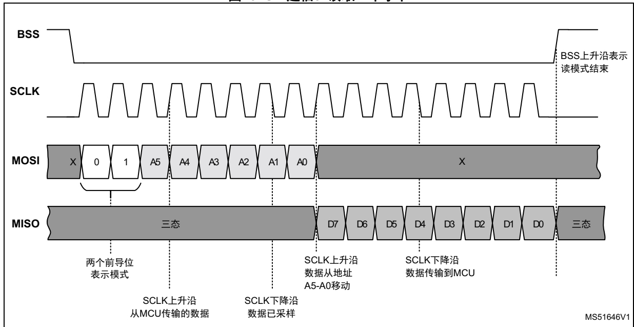
图13. SPI通信：读取一个字节
