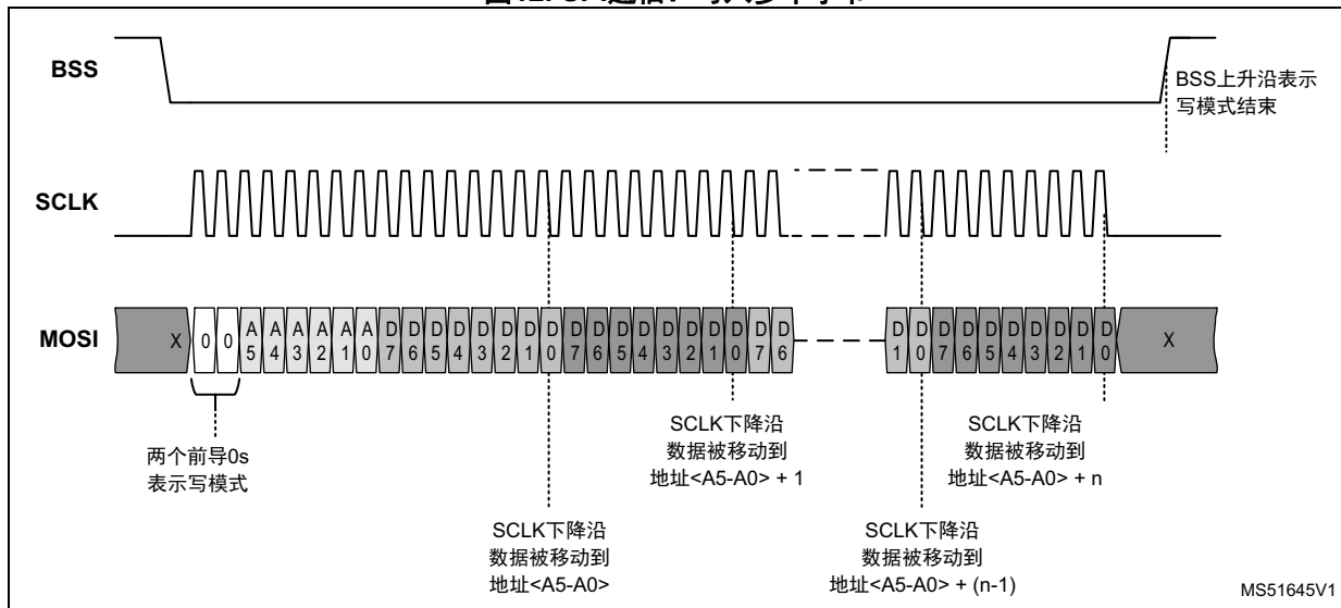
图12. SPI通信：写入多个字节
