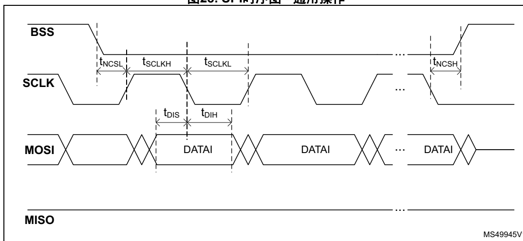
图28. SPI时序图 - 通用操作
