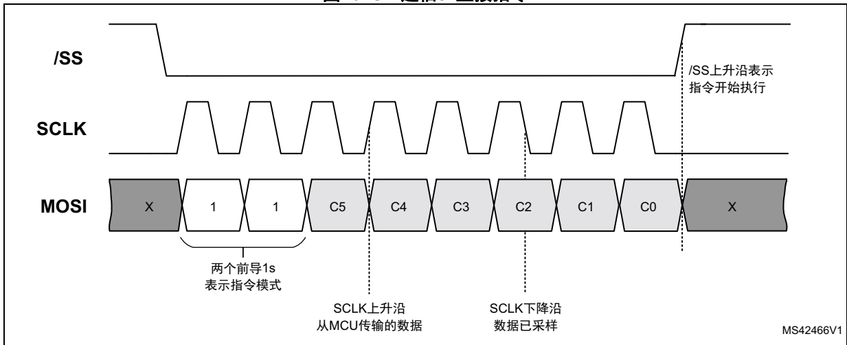
图16. SPI通信：直接指令
