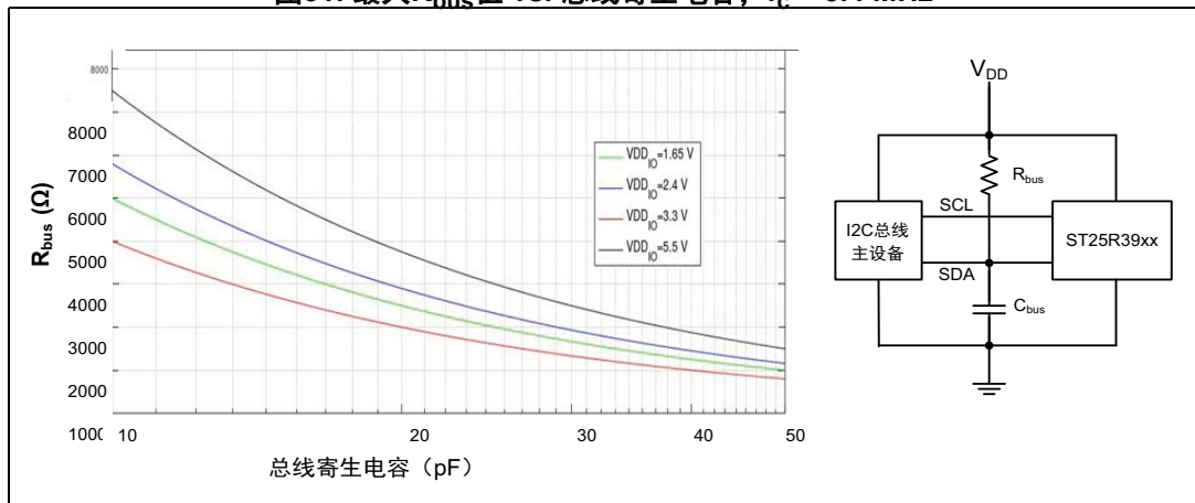
图31. 最大 R_{bus} 值 vs. 总线寄生电容, f_c = 3.4 MHz
