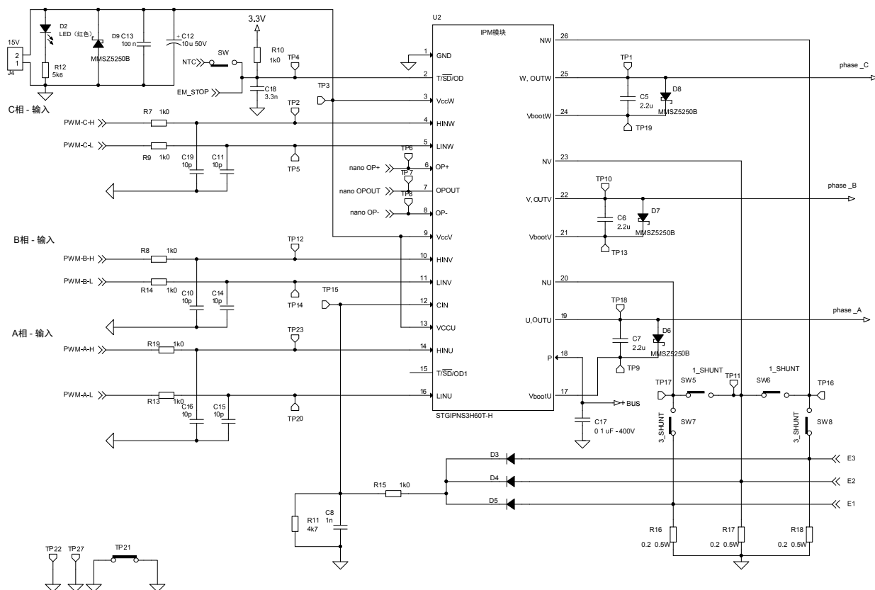
图 3. STEVAL-IPMnG3S - 电路原理图 (图 3, 共 5 图)
