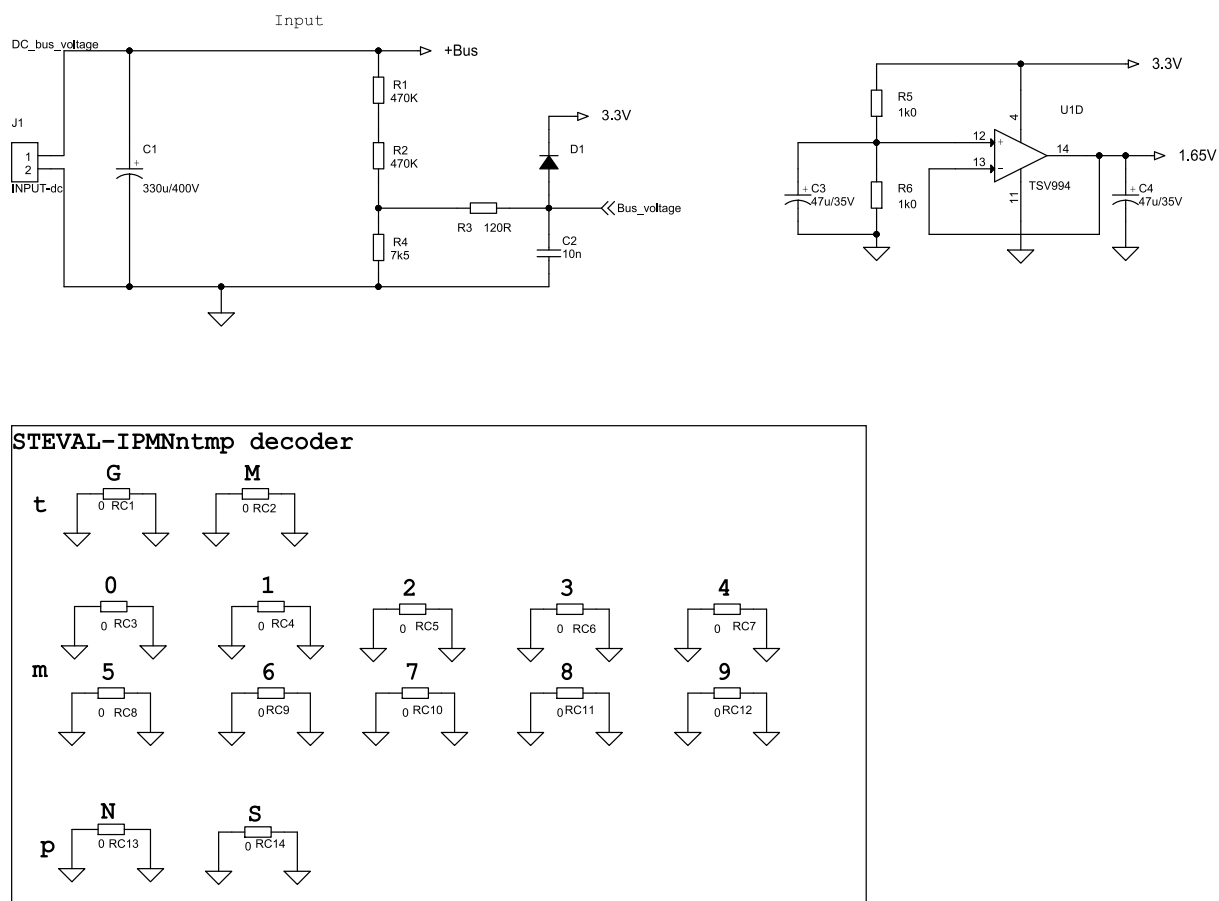
图 1. STEVAL-IPMnG3S - 电路原理图（图 1，共 5 图）
