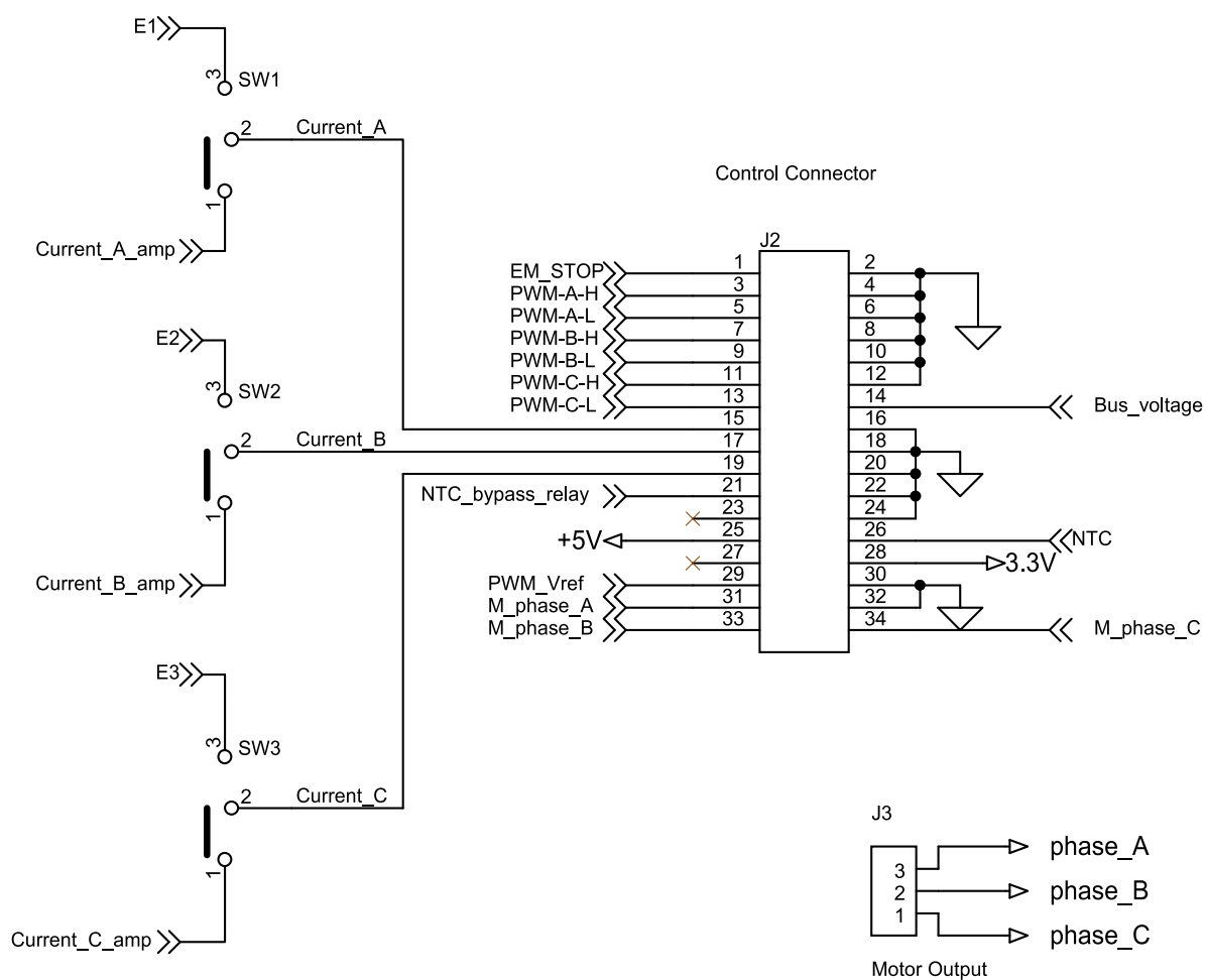
图 2. STEVAL-IPMnG3S - 电路原理图 (图 2, 共 5 图)
