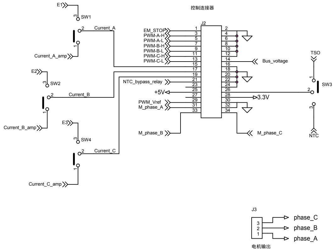
图 2. STEVAL-IPM10B 电路原理图 (图 2, 共 6 图)
