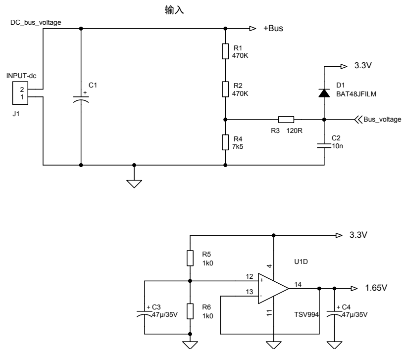
图 3. STEVAL-IPM10B 电路原理图 (图 3, 共 6 图)
