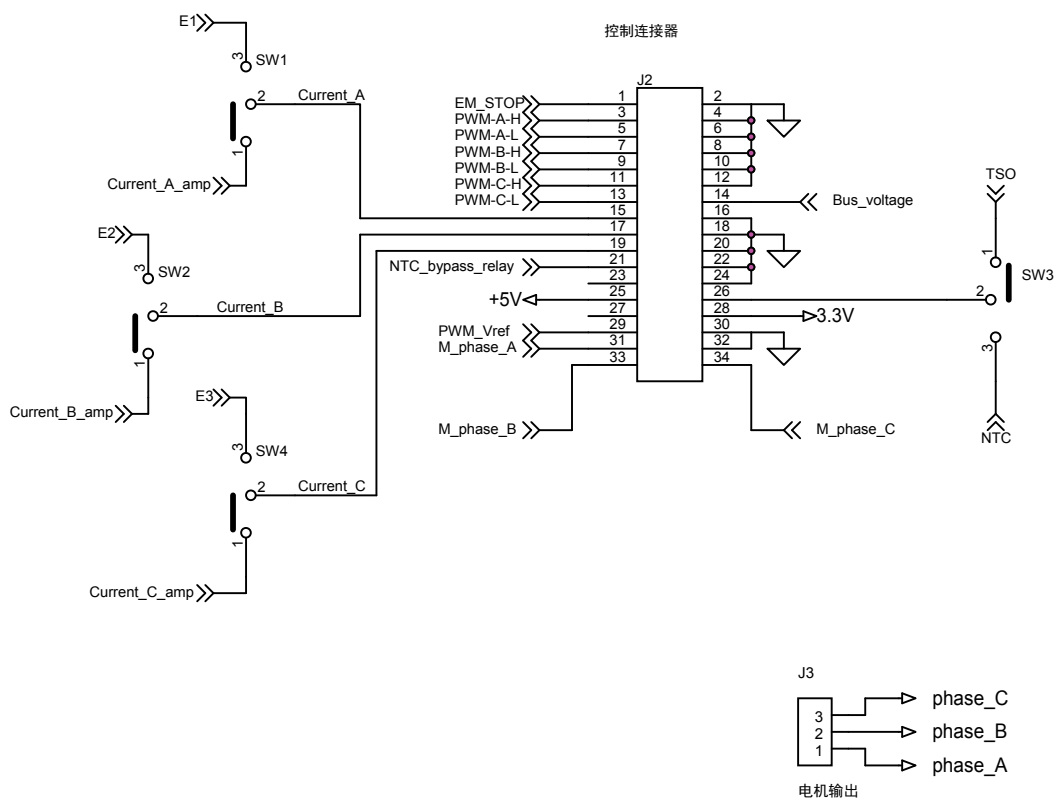
图 2. STEVAL-IPM08B 电路原理图 (图 2, 共 6 图)
