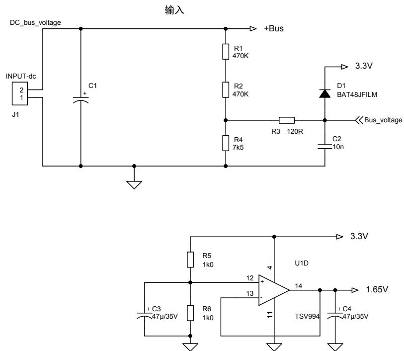
图 3. STEVAL-IPM07F 电路原理图 (图 3, 共 6 图)
