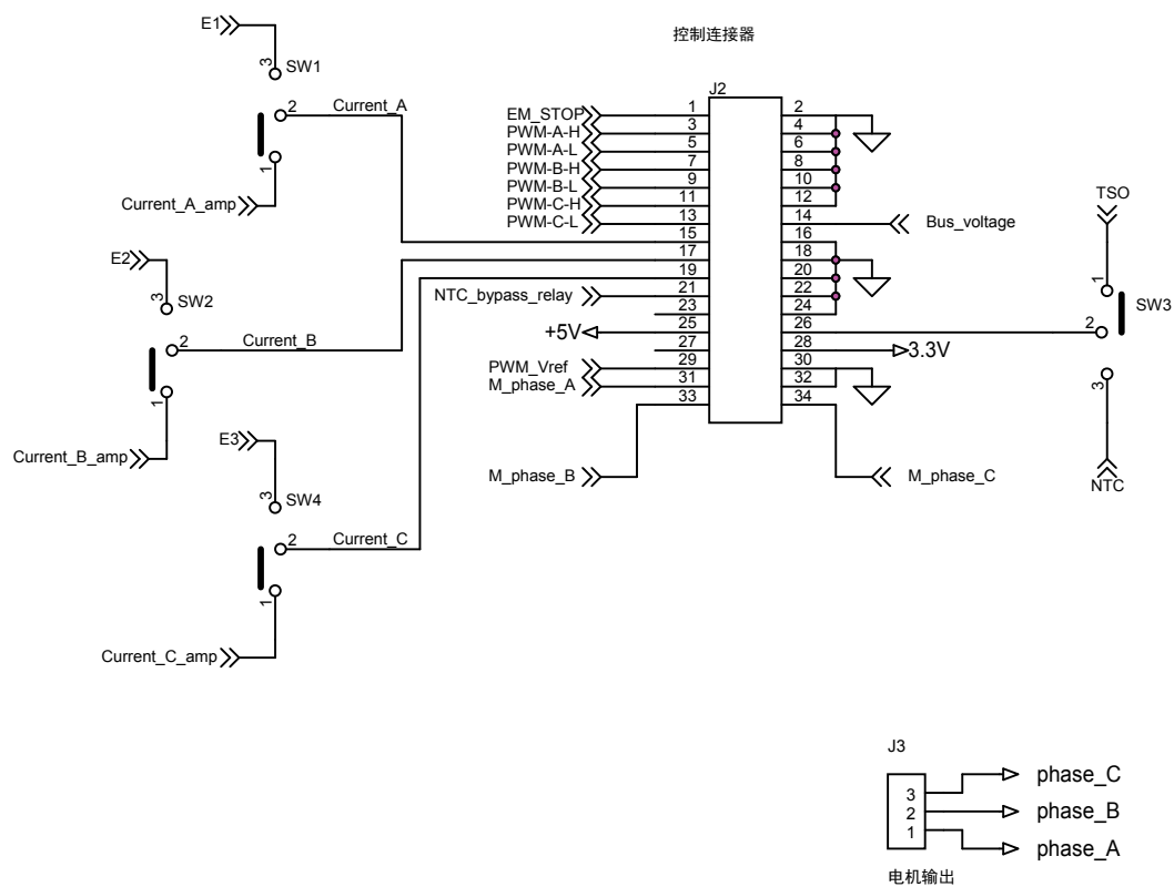
图 2. STEVAL-IPM07F 电路原理图 (图 2, 共 6 图)
