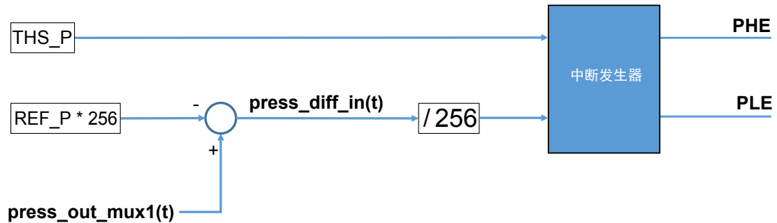
图 7. 中断发生器
