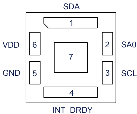
图 1. 引脚连接（底视图）
