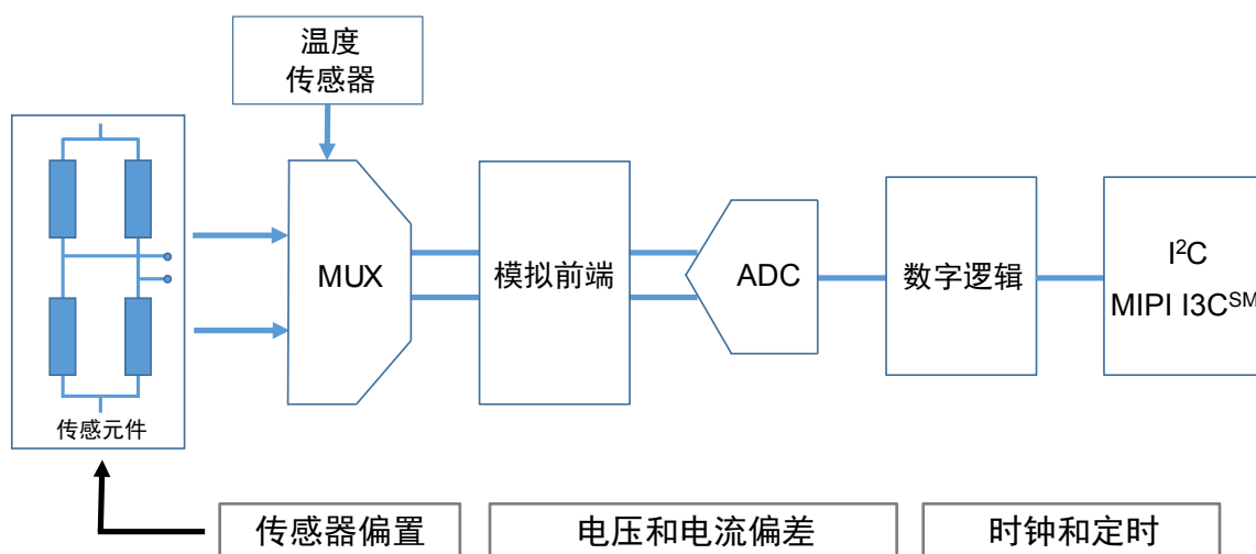
图 4. LPS28DFW 架构框图
