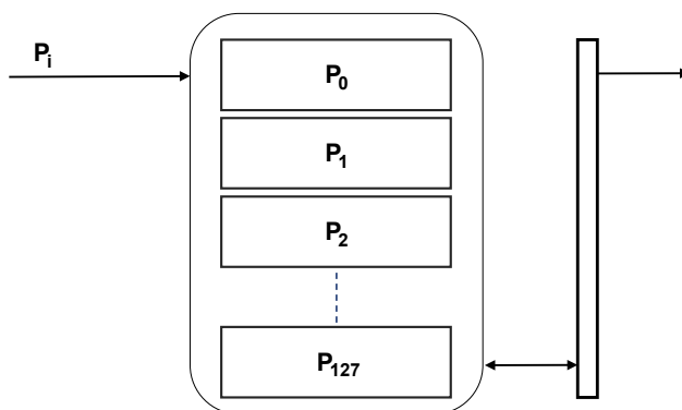
图 16. 使能了达到水印值时停止功能的 FIFO 模式
