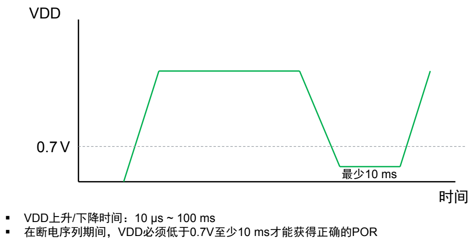
图 2. VDD 开机/关机时序
