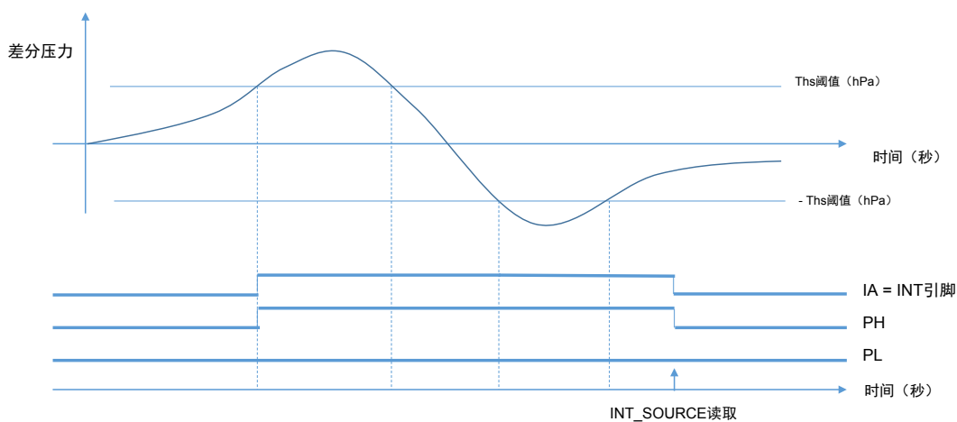
图 12. 锁存使能 ( LIR = 1 )：中断行为
