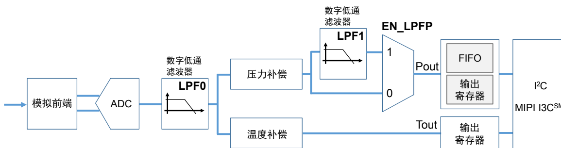
图 5. LPS28DFW 数字 LP 滤波器框图
