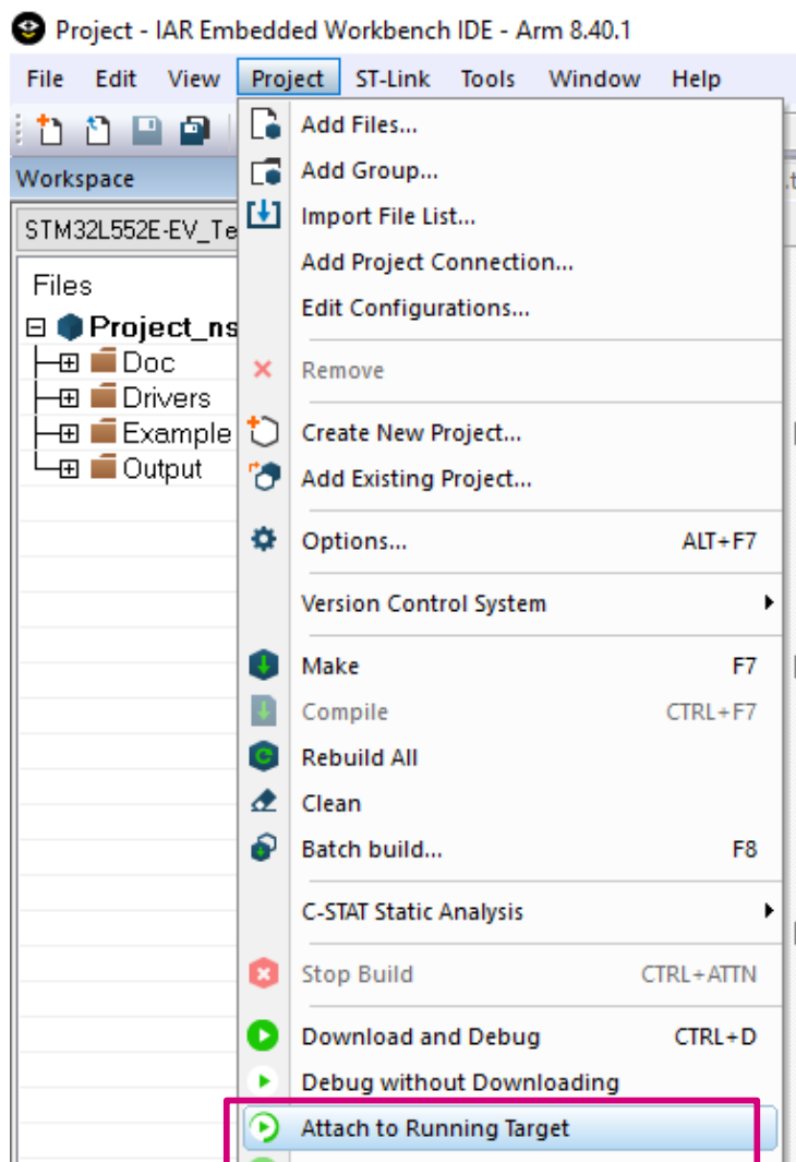
图 50. 附加于运行中的目标选项
