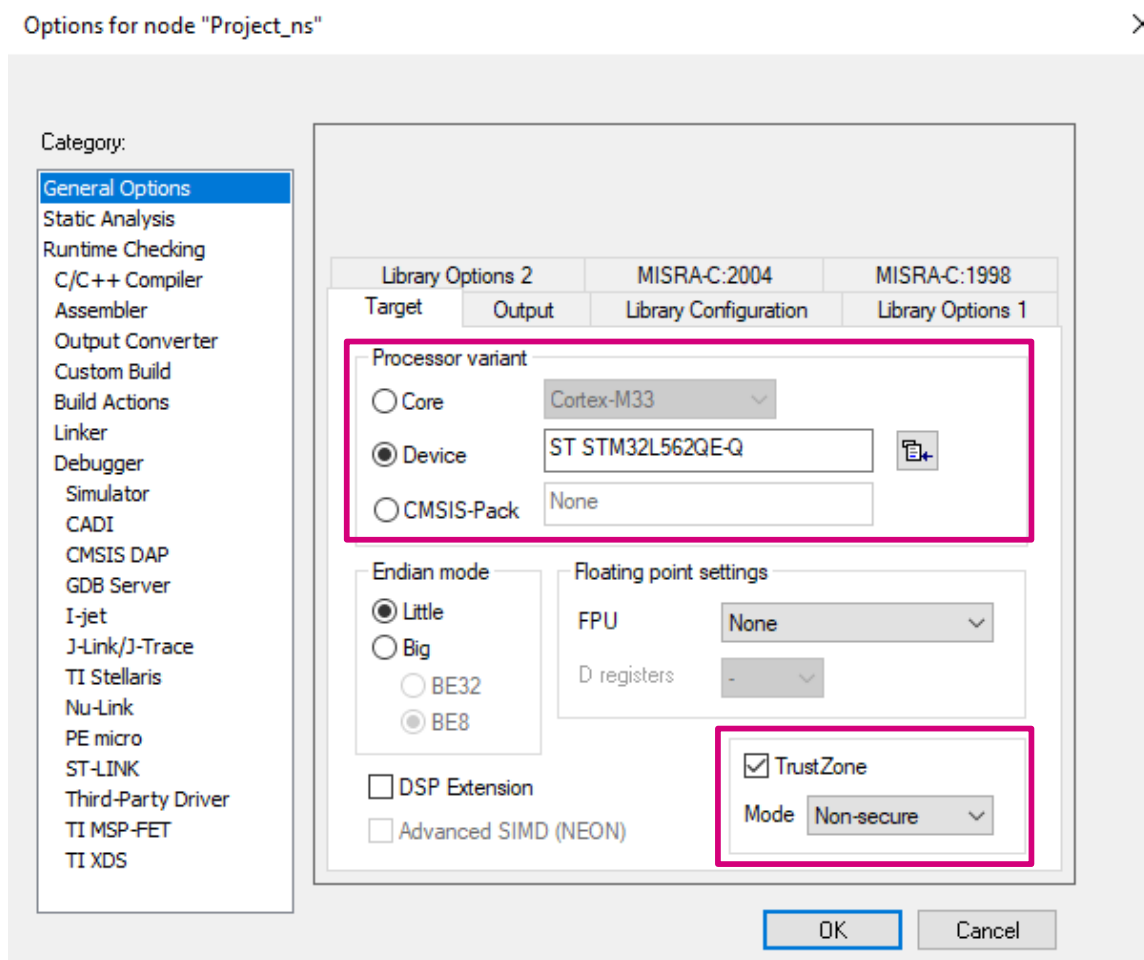
图 38. 项目设置：一般选项
