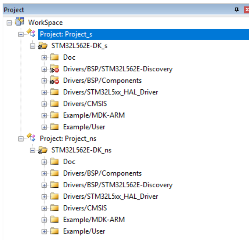
图 5. MDK-ARM 项目结构
