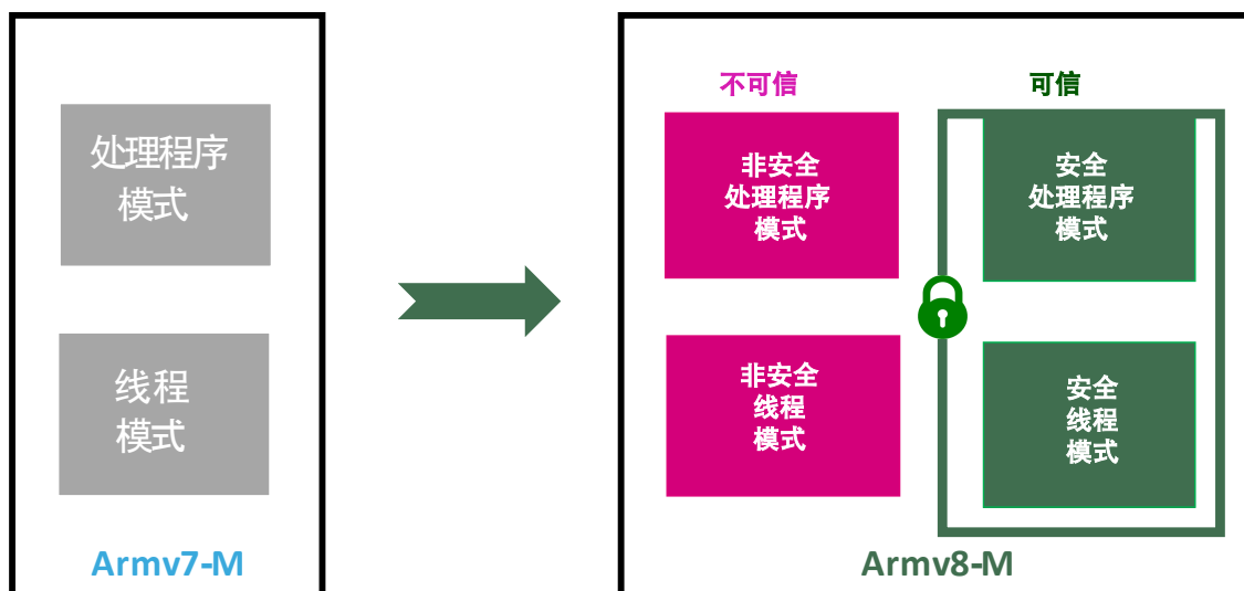
图 1. Armv8-M 中的安全状态
