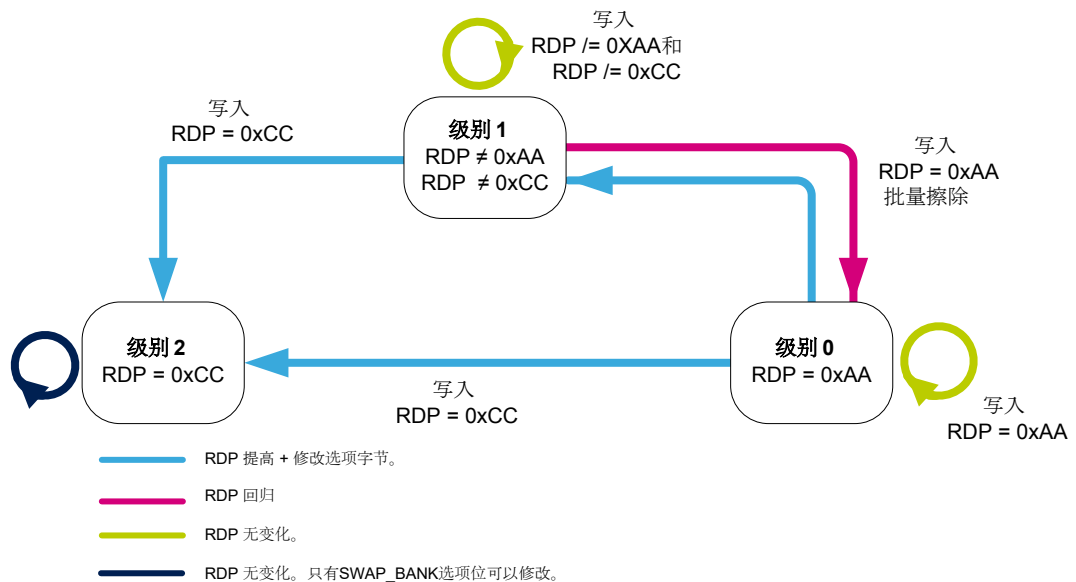
图 2. TrustZone®被禁用（TZEN = 0）后的 RDP 级别转换流程
