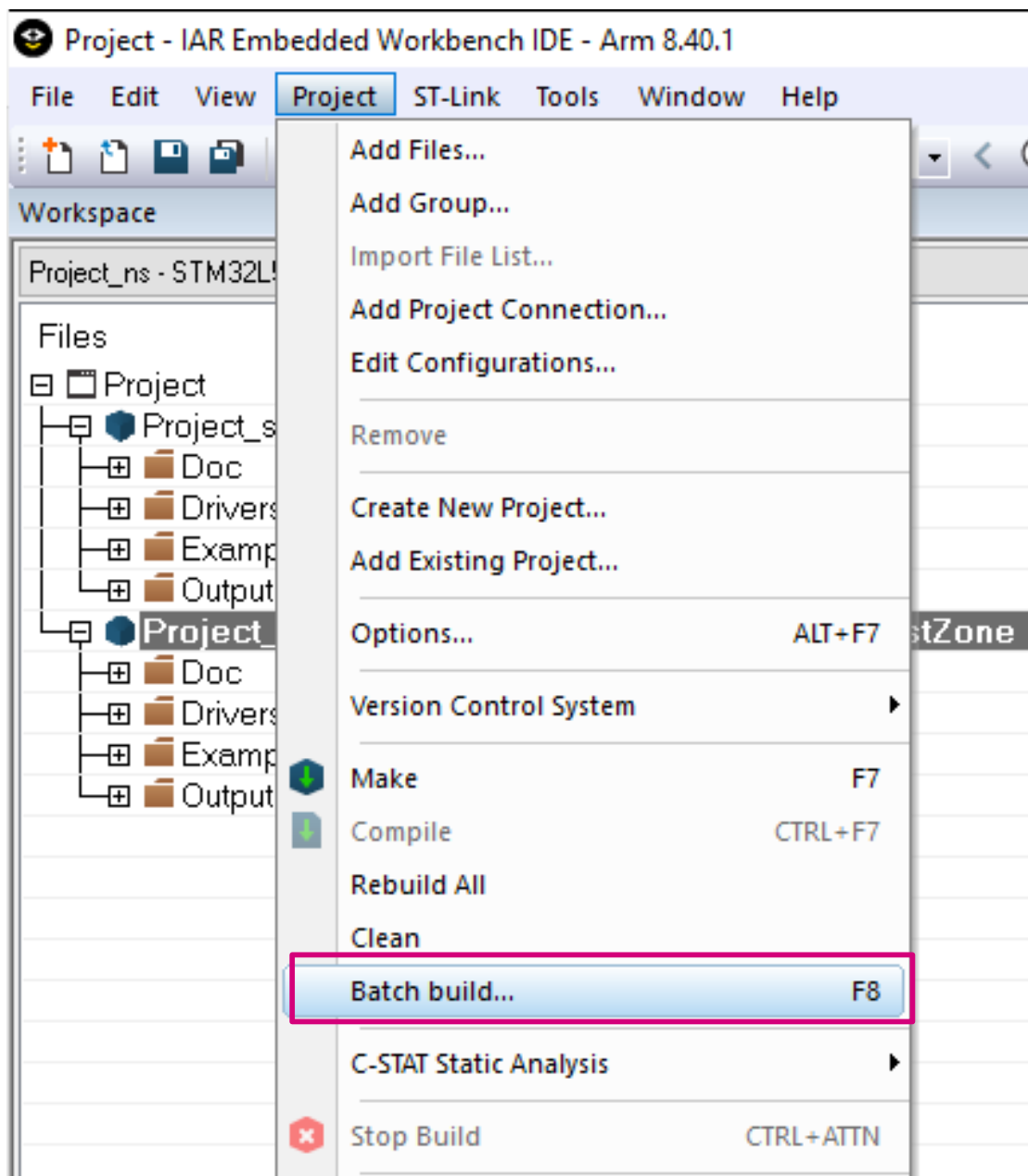
图 41. 项目批编译
