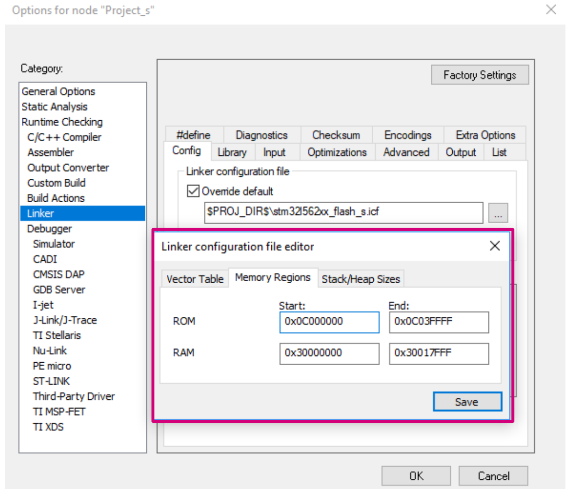
图 33. 链接器配置
