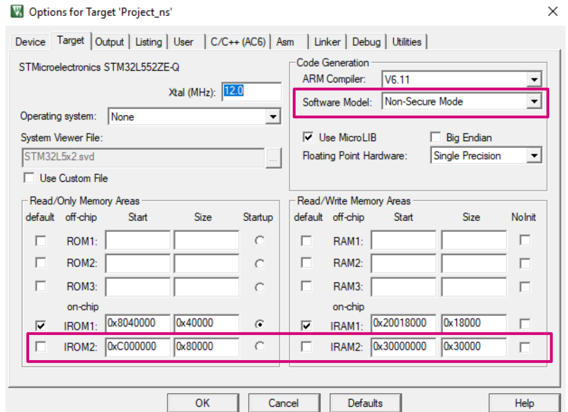
图 16. 内存配置
