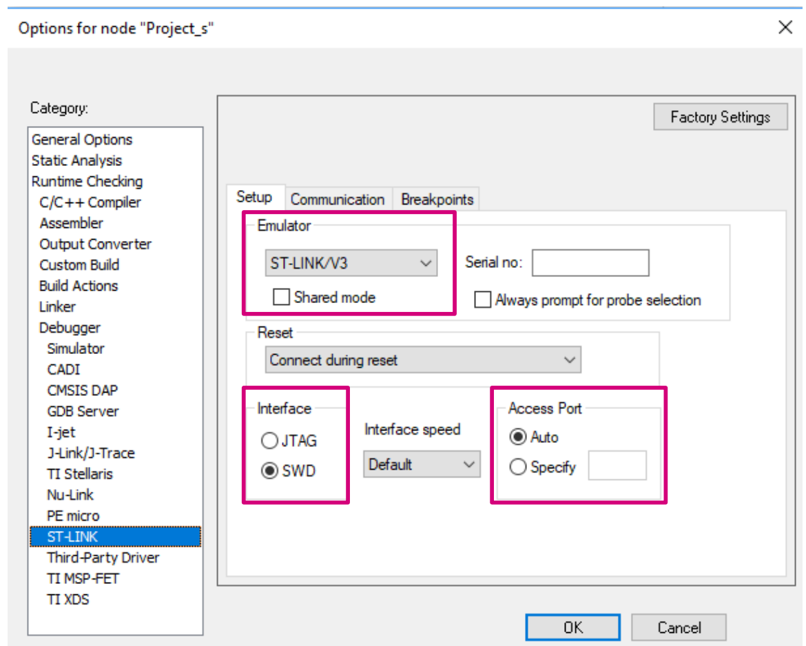
图 37. 项目设置
