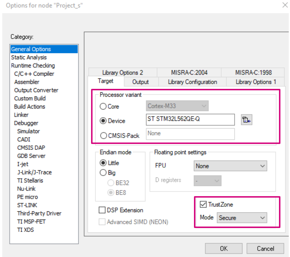
图 32. 设备选择
