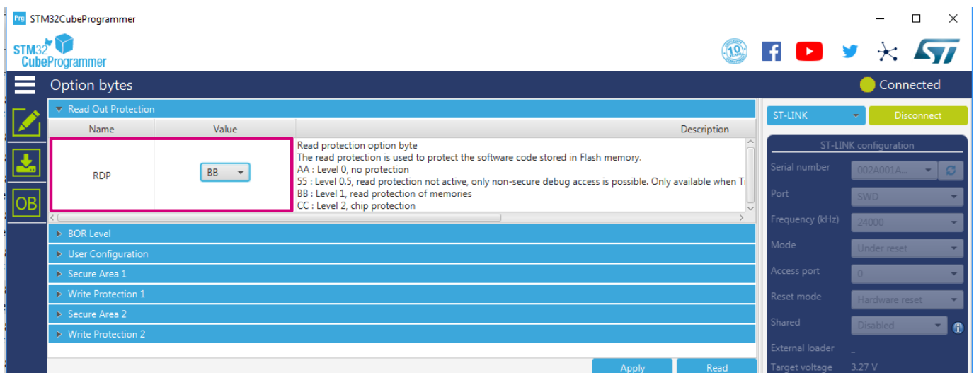
图 48. RDP=0.5
