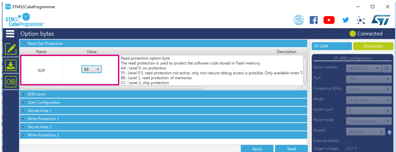
图 47. 使用 STM32CubeProgrammer v2.2.0 配置选项字节
