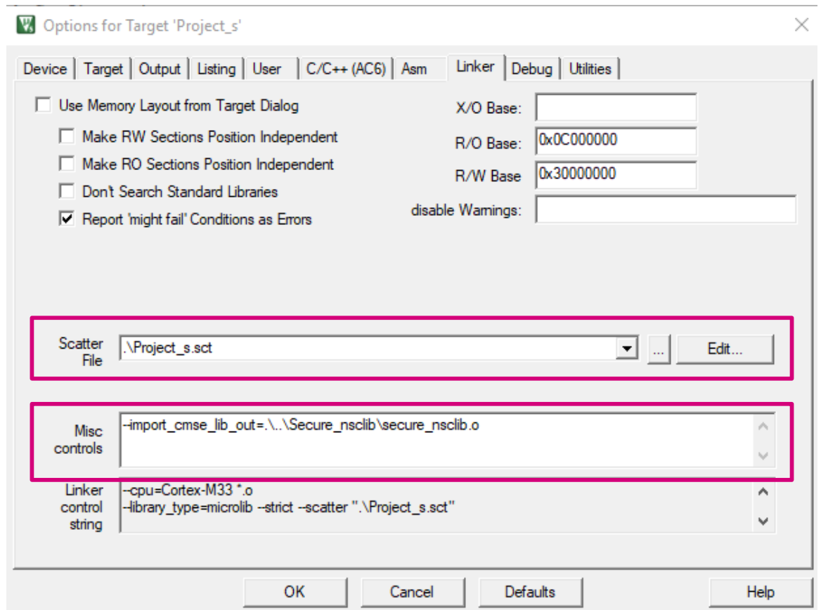
图 9. Project_s 链接器配置
