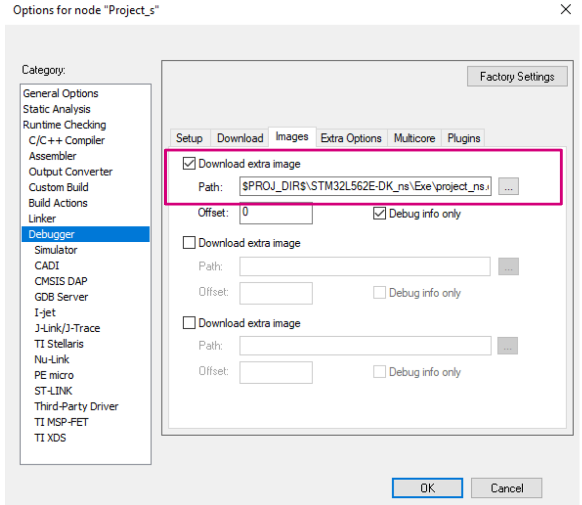
图 36. 选择非安全输出文件作为额外映像
