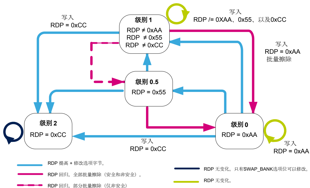
图 3. TrustZone® 被禁用 (TZEN = 1) 后的 RDP 级别转换流程
