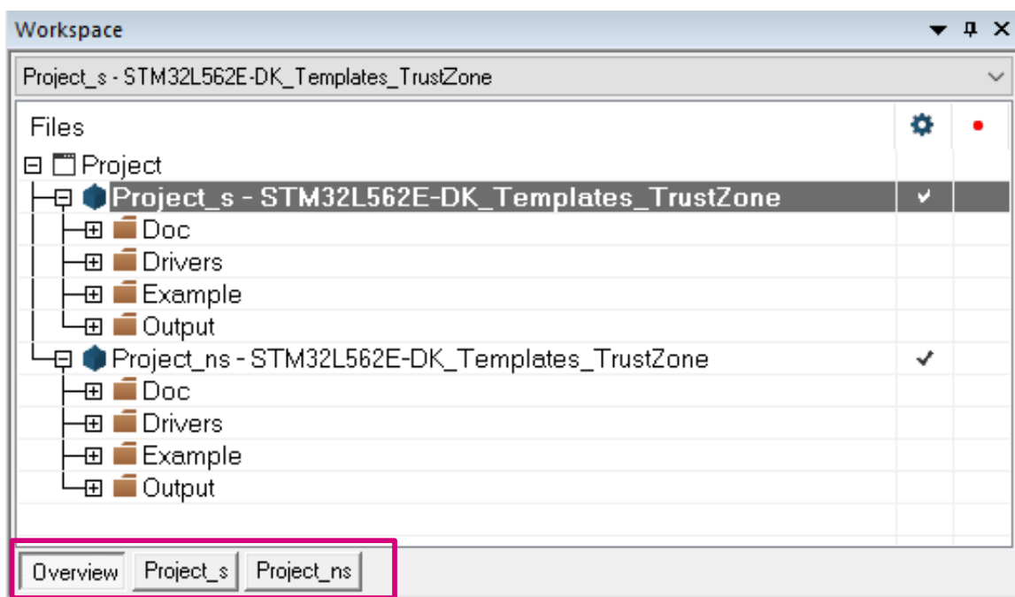
图 30. EWARM v8.40.1 项目浏览器视图
