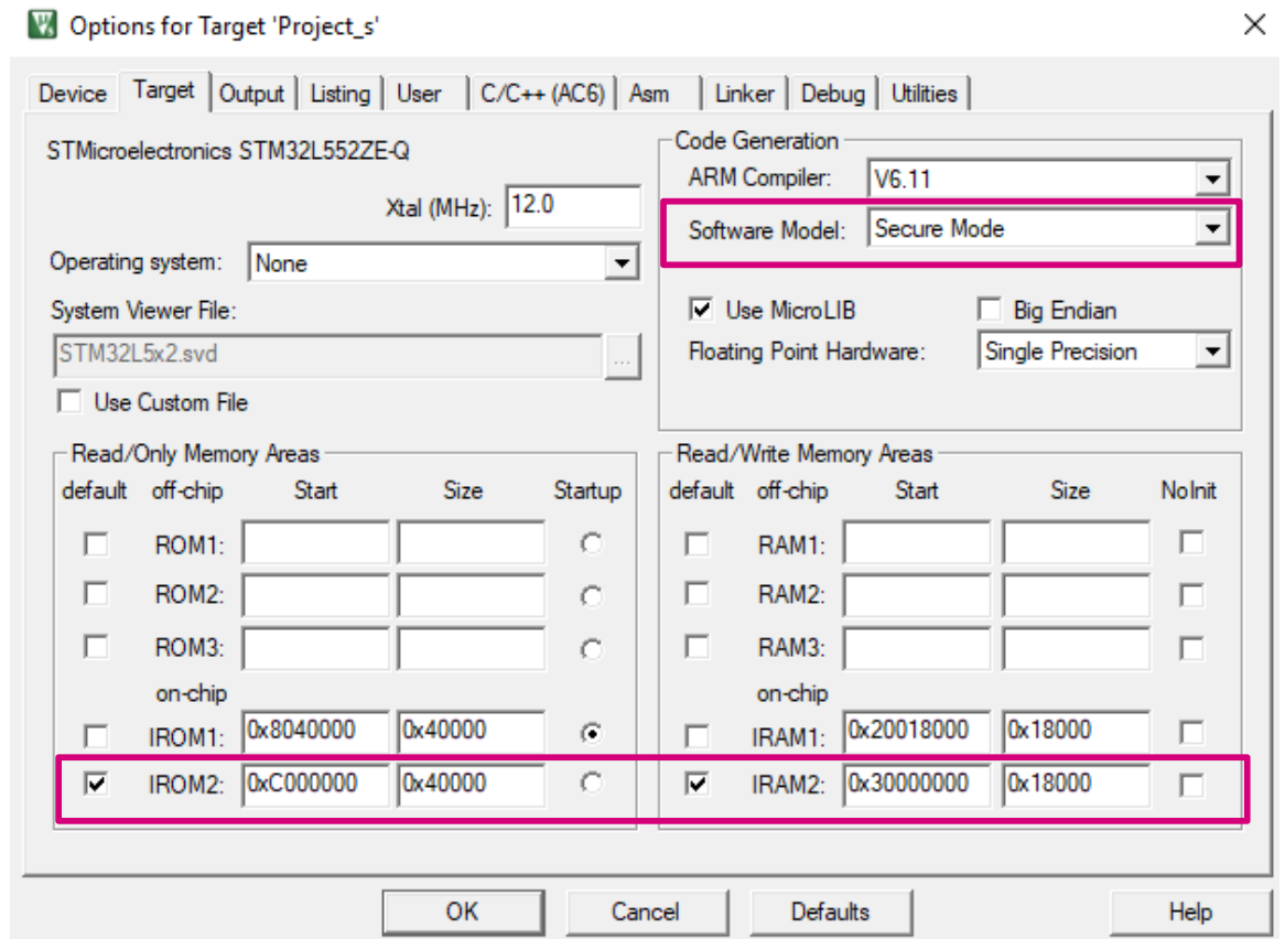
图 8. Project_s 目标选项
