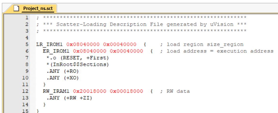
图 18. 分散加载文件示例
