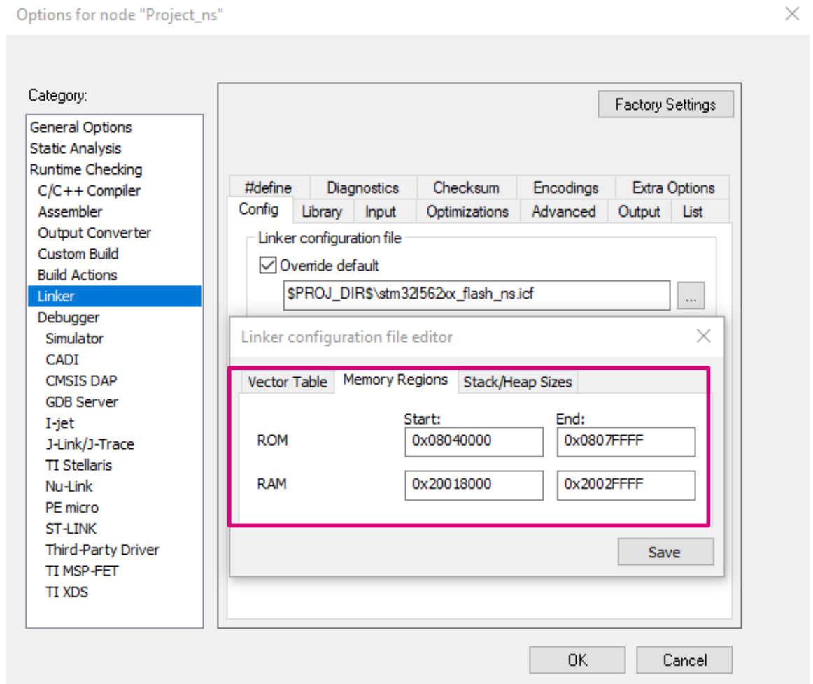
图 39. 项目链接器配置
