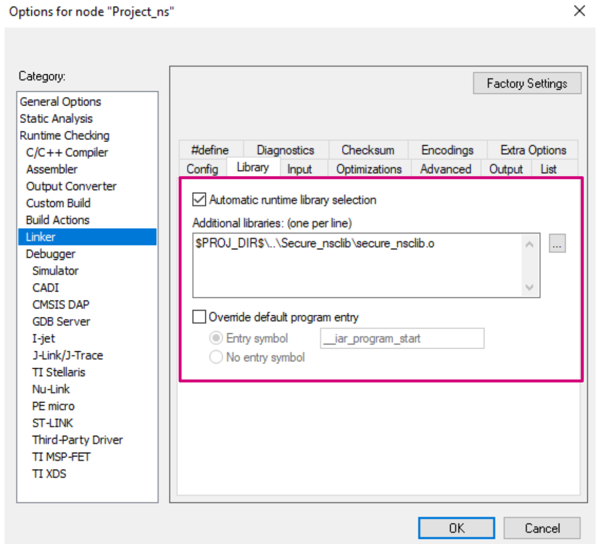
图 40. 链接器库设置
