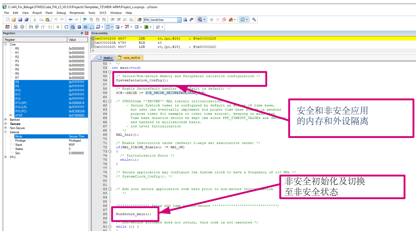
图 27. Main.c 示例代码
