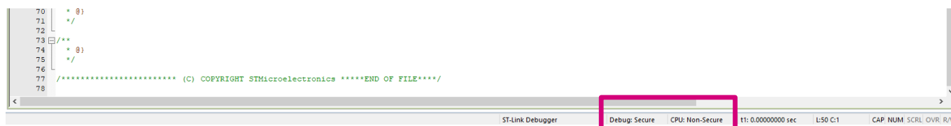
图 29. CPU 状态
