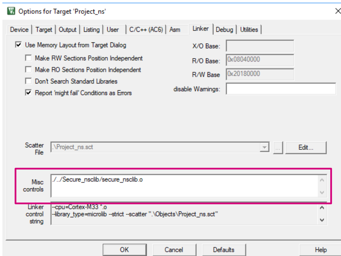
图 17. 链接器选项
