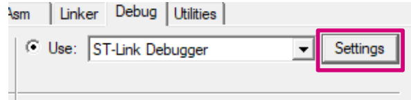
图 19. 调试设置
