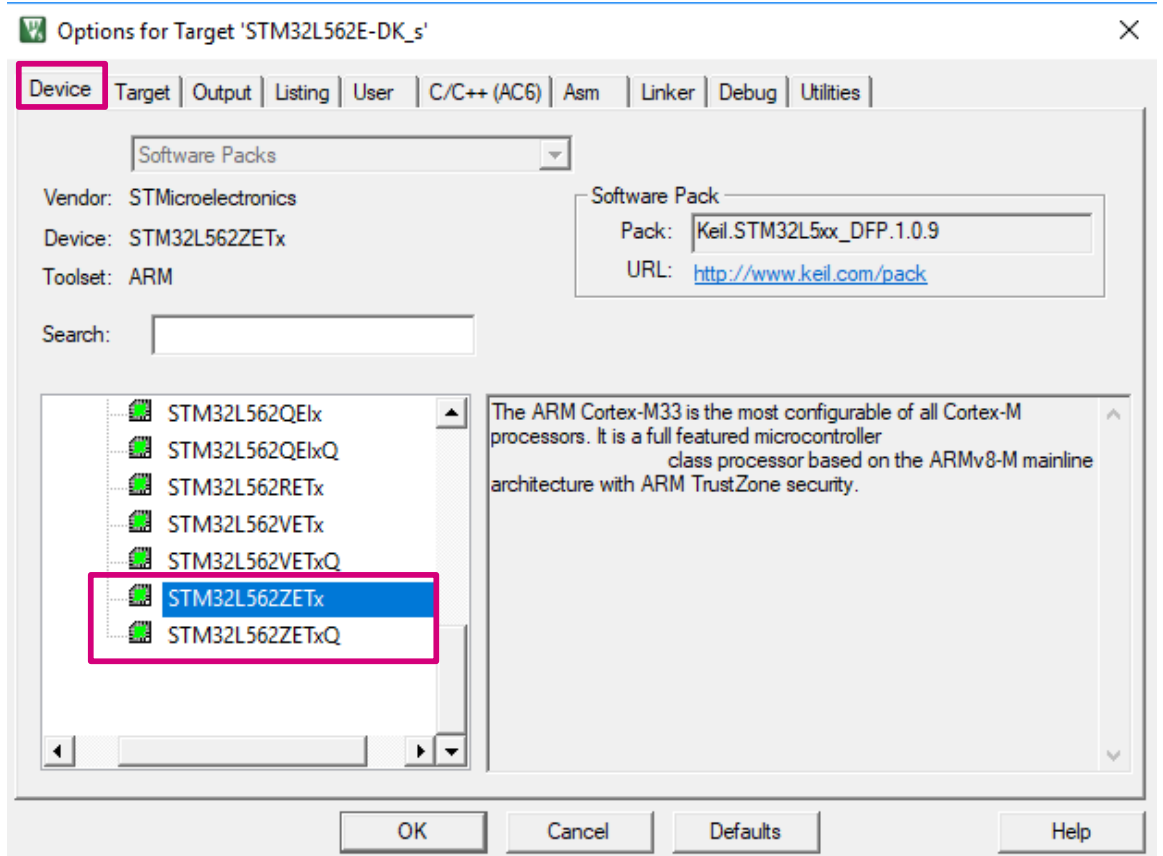
图 15. 设备选择
