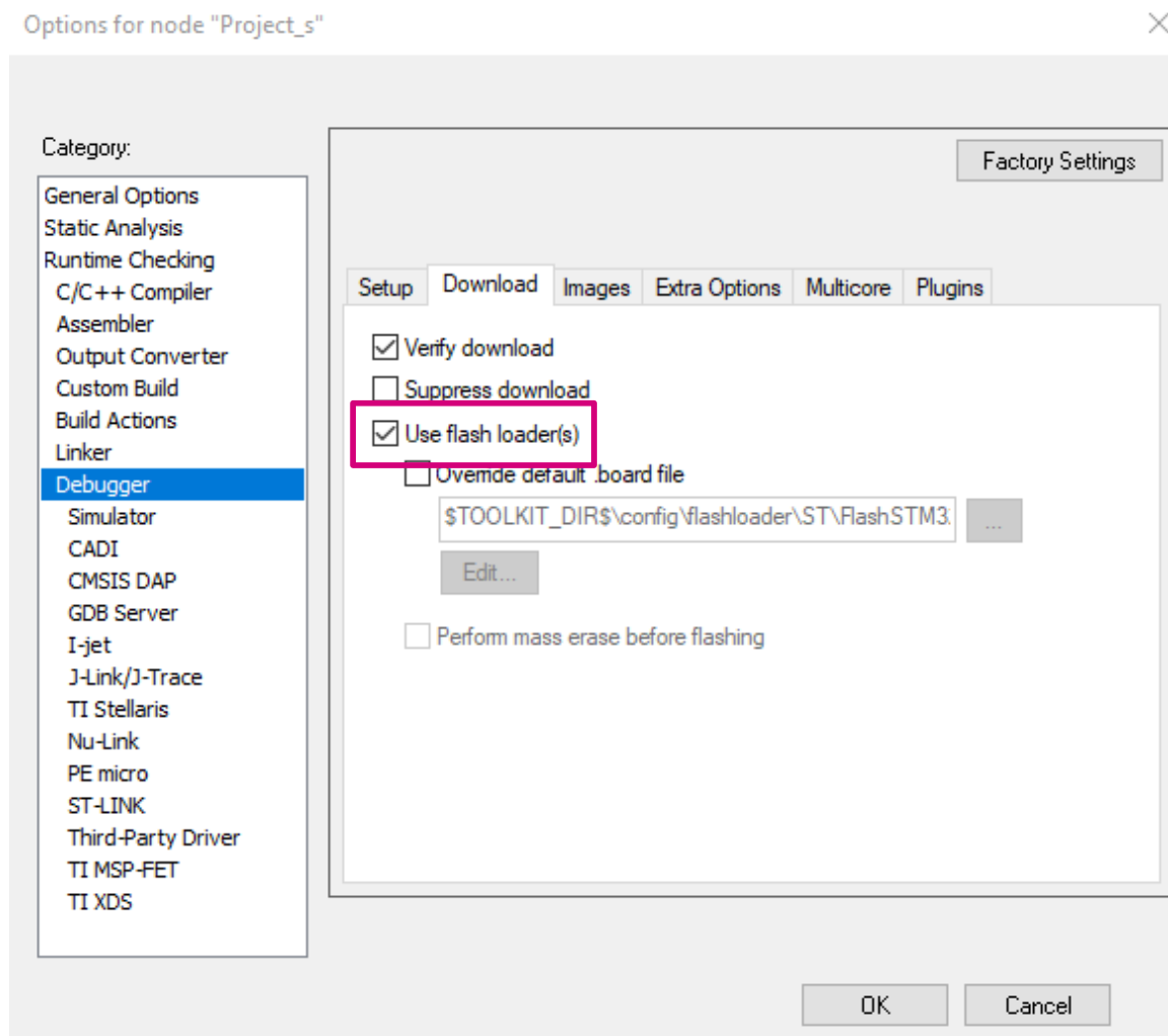
图 35. FlashLoader 选择
