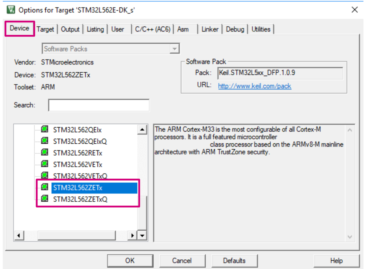
图 7. 设备选择
