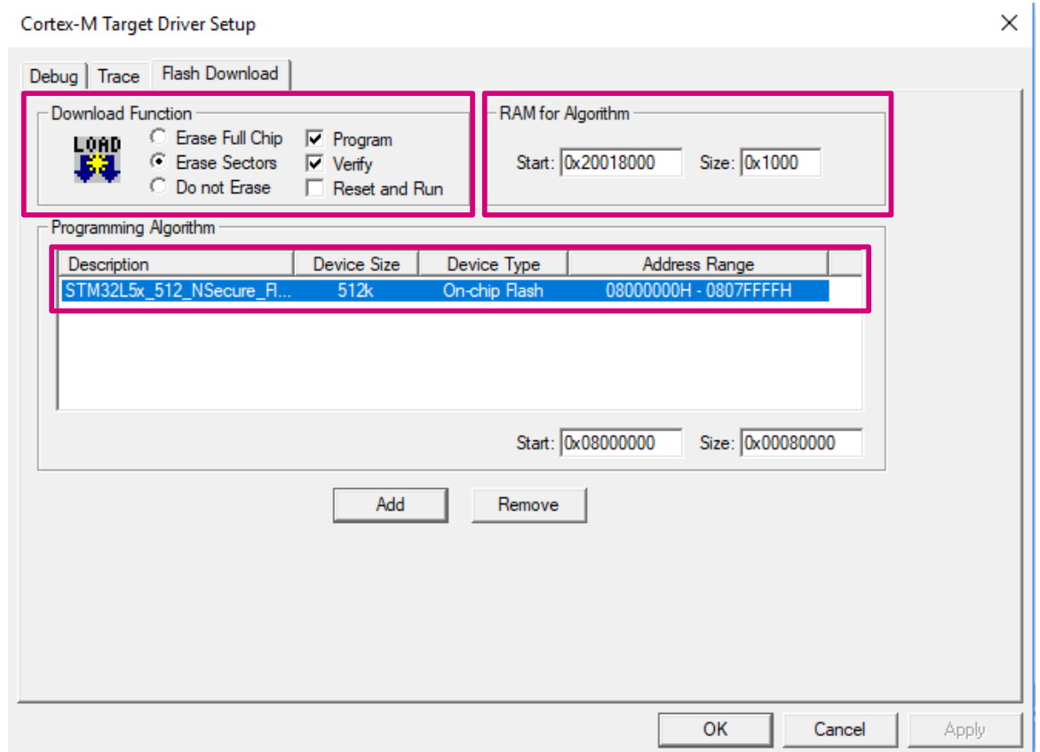
图 20. FlashLoader 配置
