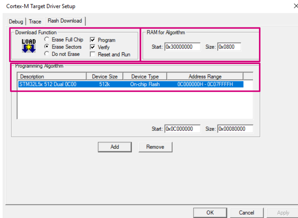
图 13. 闪存加载程序设置
