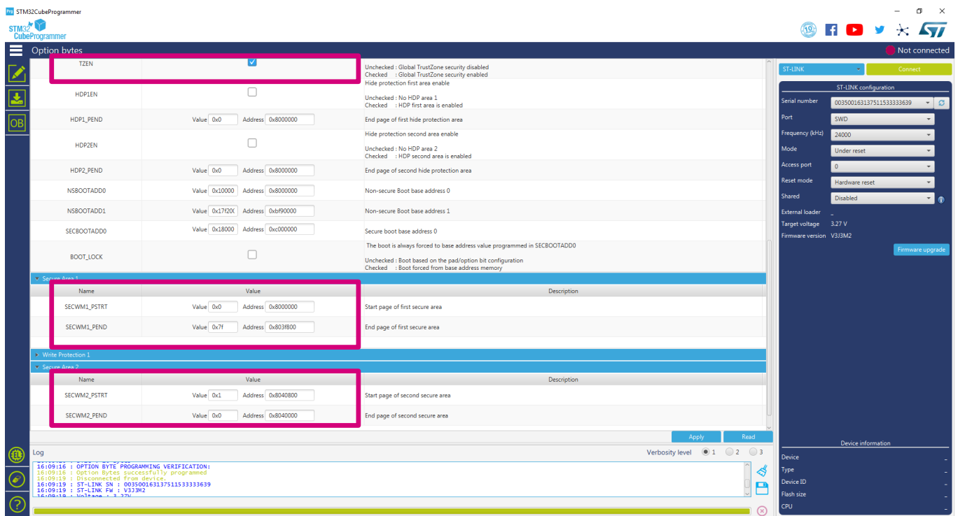
图 4. 使用 STM32CubeProgrammer 配置选项字节
