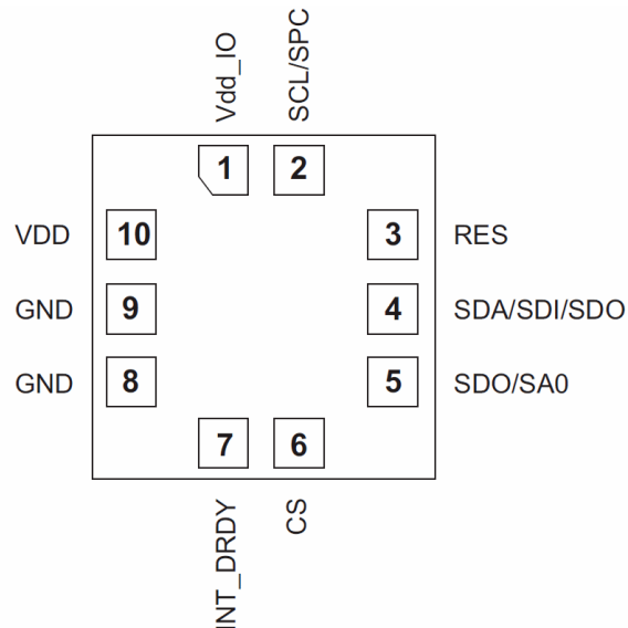
图 1. 引脚连接
