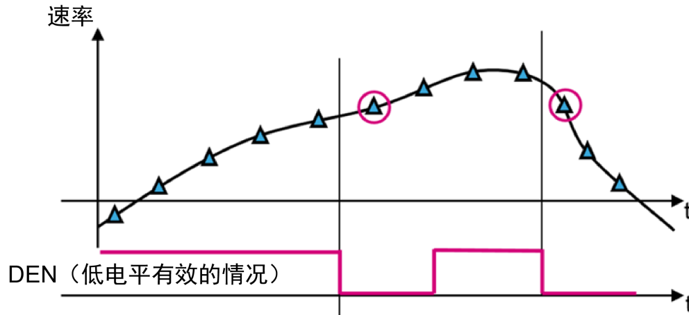
图 7. 边沿感应触发模式，DEN 低电平有效
