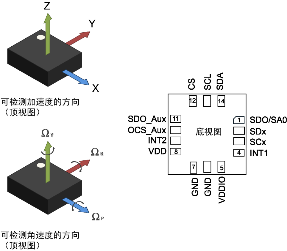
图 1. 引脚连接
