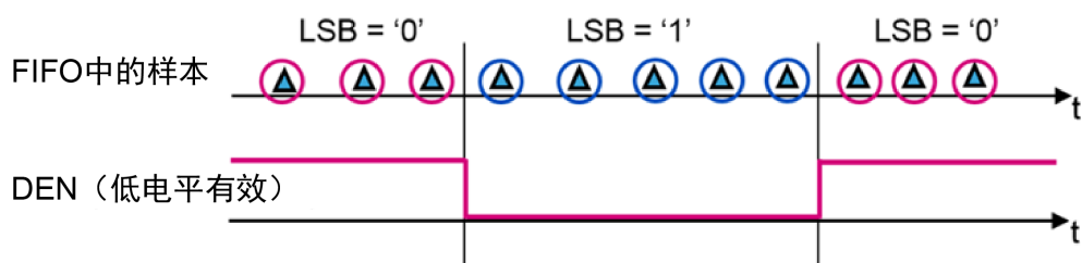
图 9. 电平感应触发模式，DEN 低电平有效
