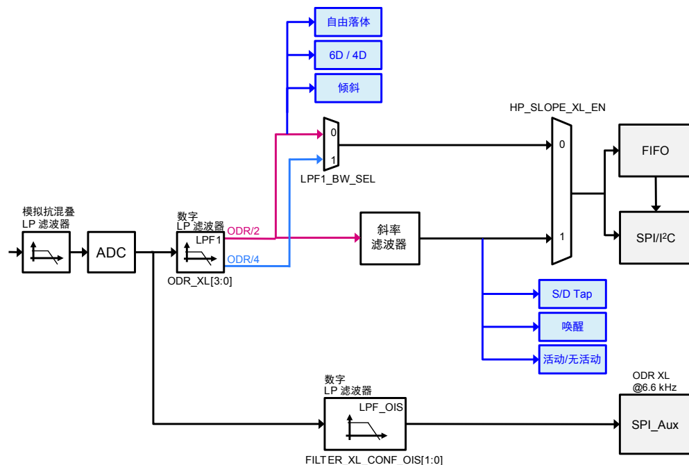
图 3. 加速度计滤波链（模式 4）
