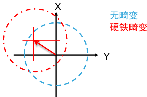
图 25. 硬铁效应（X-Y 2D 散点图）
