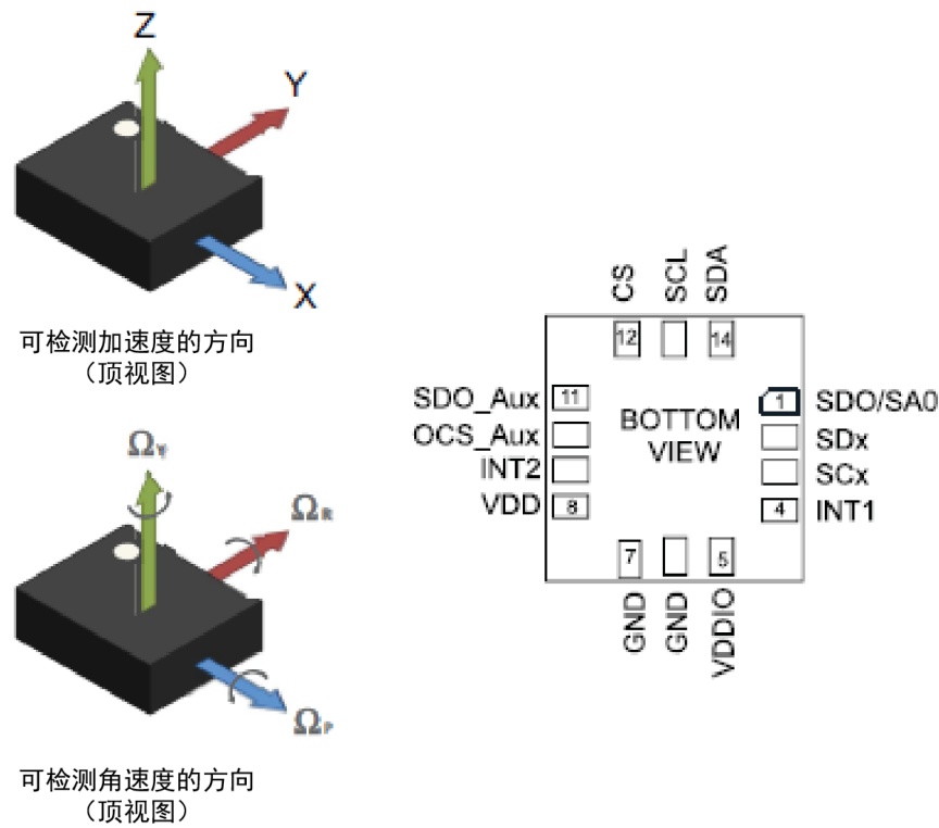
图 1. 引脚连接
