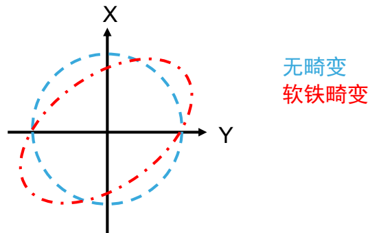
图 26. 软铁效应 (X-Y 2D 散点图)
