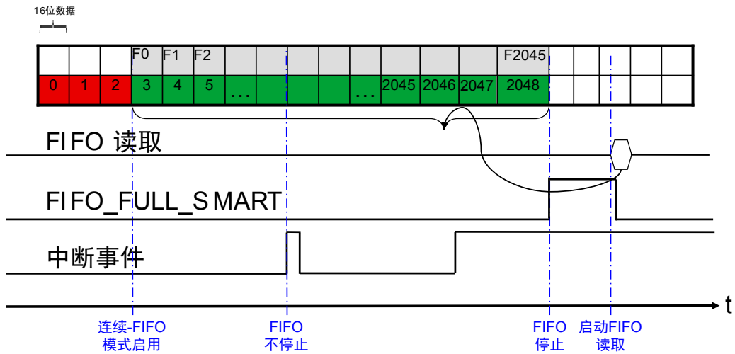
图 31. 连续-FIFO 模式
