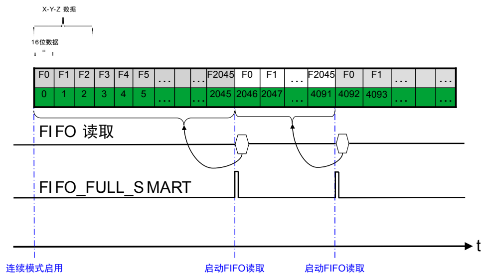
图 30. 连续模式
