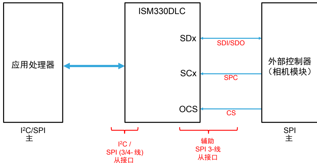
图 28. 模式 3/4 下的外部控制器连接 (SPI 3 线)
