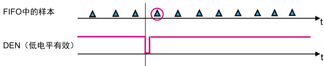
图 11. 电平感应锁存模式，DEN 低电平有效
