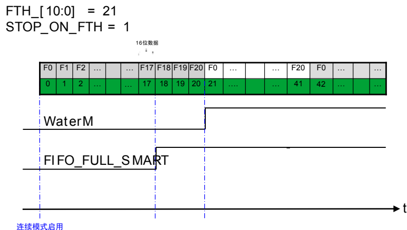
图 36. 连续模式下的 FIFO 阈值 ( STOP\_ON\_FTH=1 )
