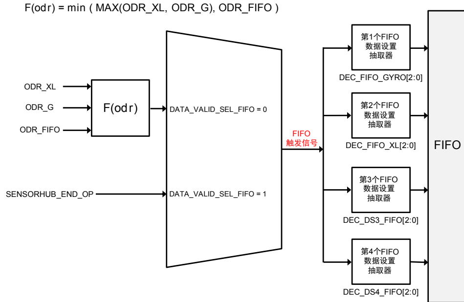
图 33. FIFO 触发信号选择
