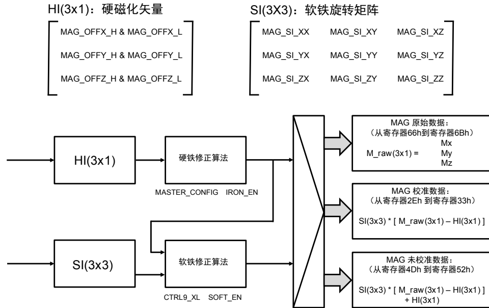
图 27. 硬铁/软铁校正框图
