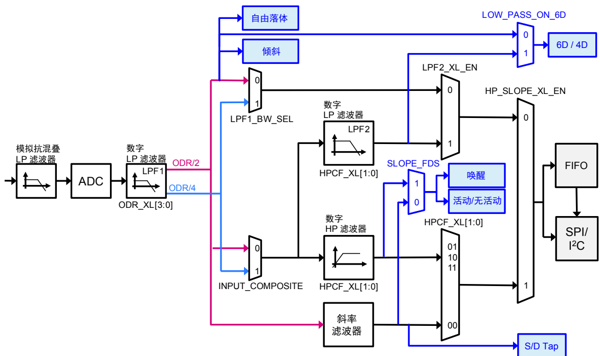
图 2. 加速度计滤波链（模式 1/2/3）
