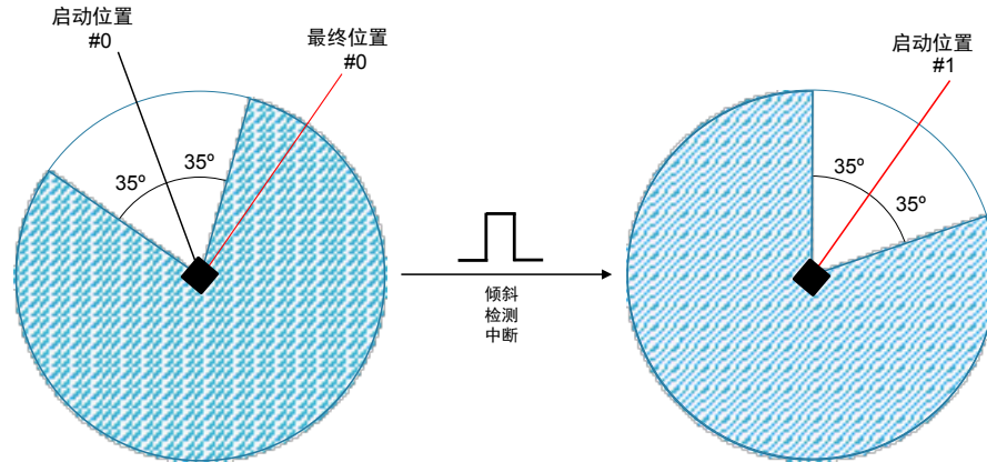
图 21. 倾斜度检测
