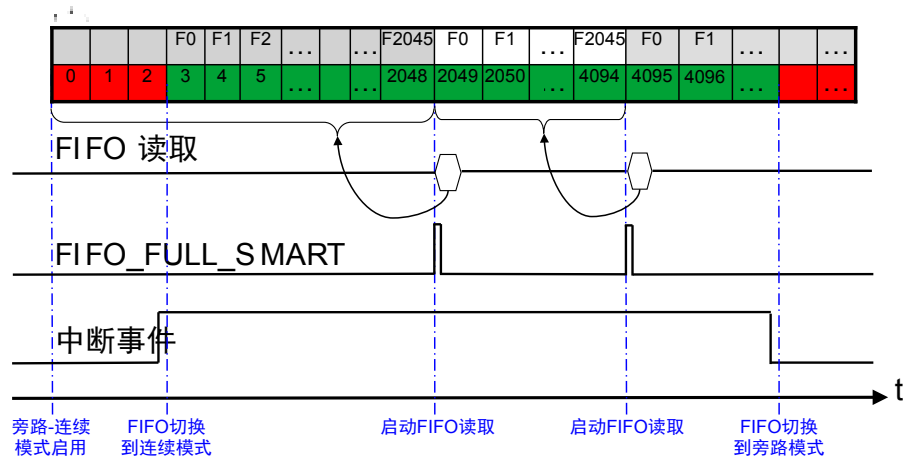
图 32. Bypass-连续模式
