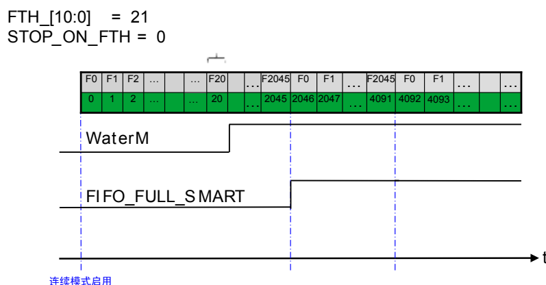
图 34. FIFO 阈值（STOP_ON_FTH=0）
