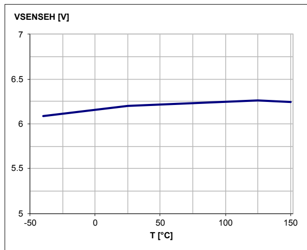
Figure 26. V_{\text{senseh}} vs T_C
