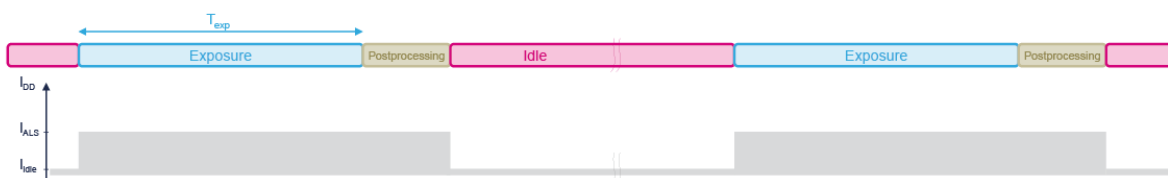
Figure 16. ALS only, single shot mode
