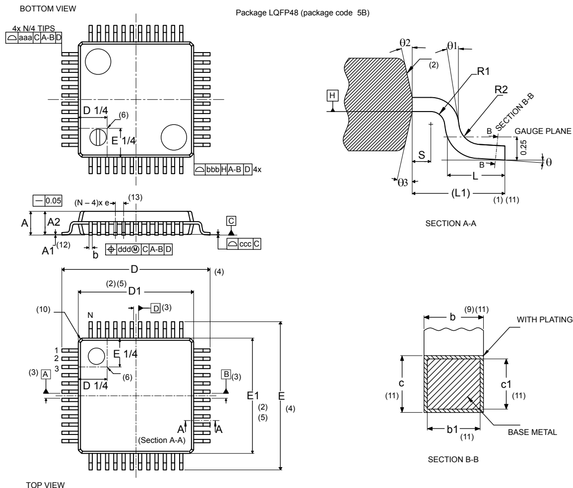
Figure 47. LQFP48- Outline (15.)
